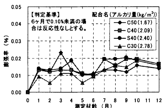
図ー8 コンクリート供試体による測定材齢と膨張量の関係
