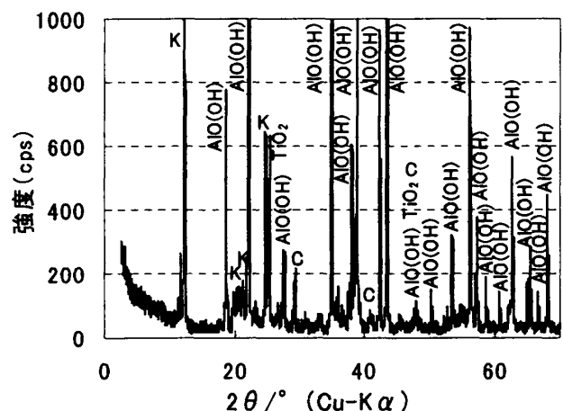
図-1 X線回折結果 (改質材：加熱前)
