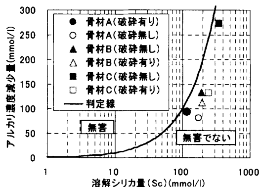
図-4 溶解シリカ量とアルカリ濃度減少量の関係
