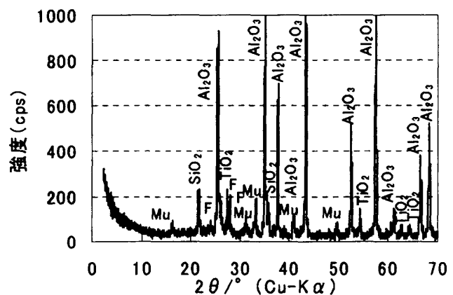
図-2 X線回折結果 (改質材：加熱後)
