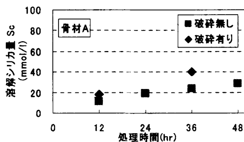
図-5 溶解シリカ量と処理時間の関係
