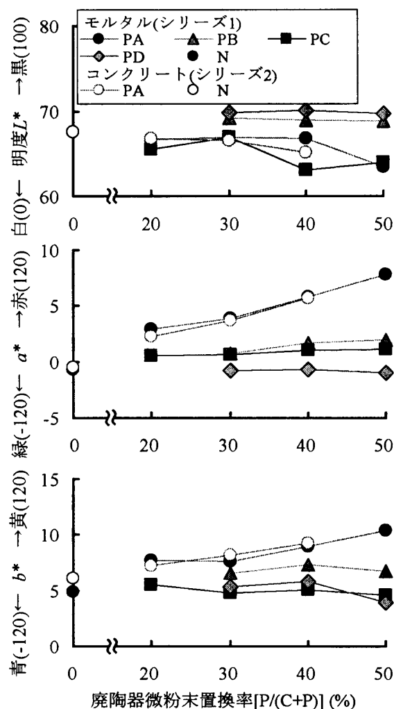
図-4 L^*a^*b^* 値と廃陶器微粉末置換率の関係
