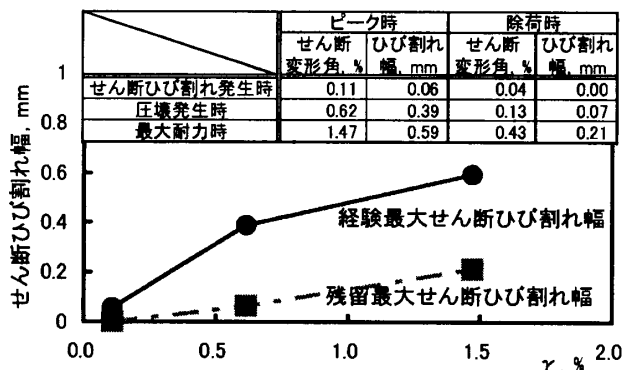
図-13 せん断変形角と損傷状況の関係
