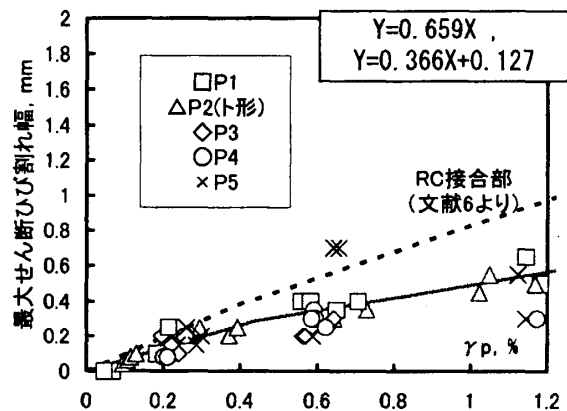
図-4 最大せん断ひび割れ幅とせん断変形角の関係
