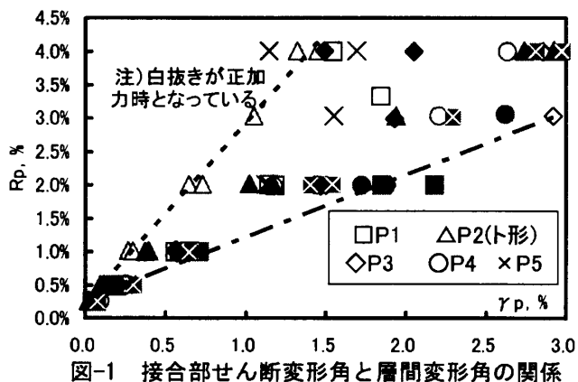
図-1 接合部せん断変形角と層間変形角の関係
