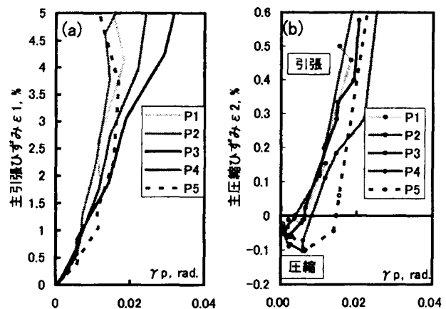
図-6 主ひずみとせん断変形角の関係
