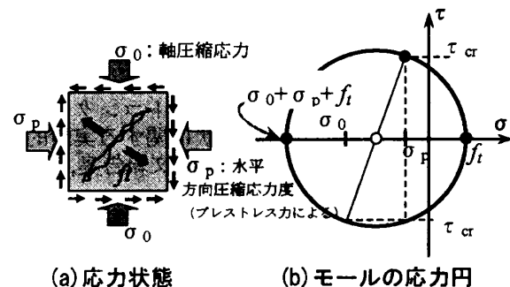
図-10 斜めひび割れ発生時の応力状態
