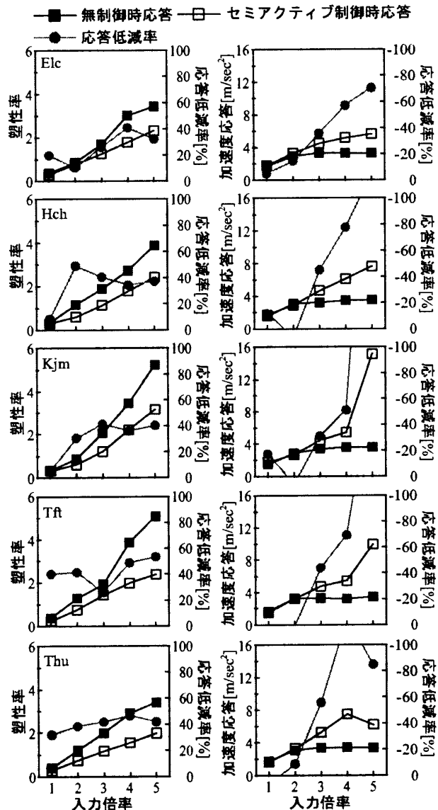
図-7 応答解析結果
