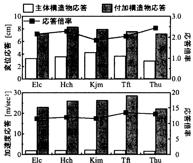
図-3 主体構造物と付加構造物比較
