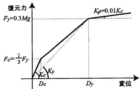
図-6 主体構造物復元力特性
