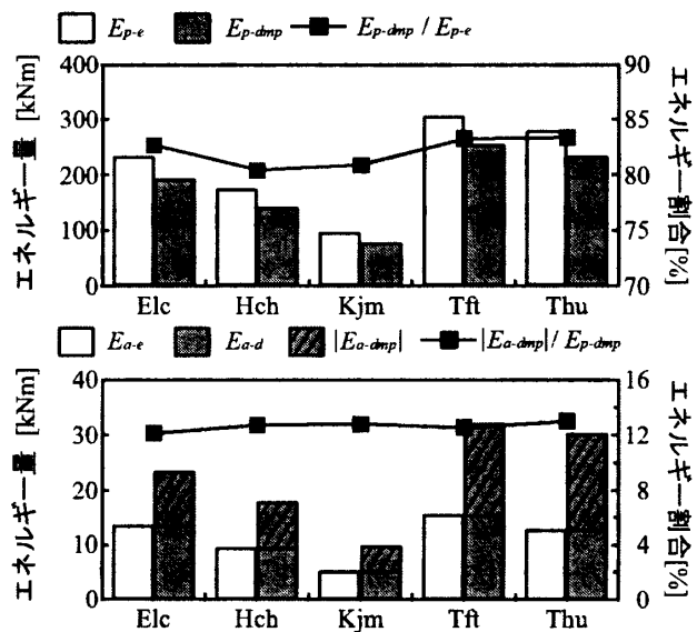
図-4 エネルギー算定結果
