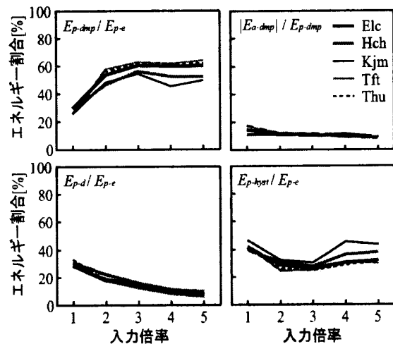
図-8 エネルギー算定結果
