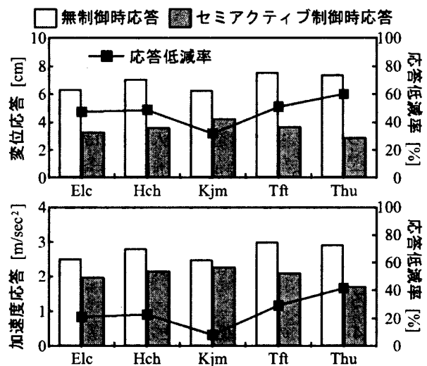
図-2 無制御時とセミアクティブ制御時比較
