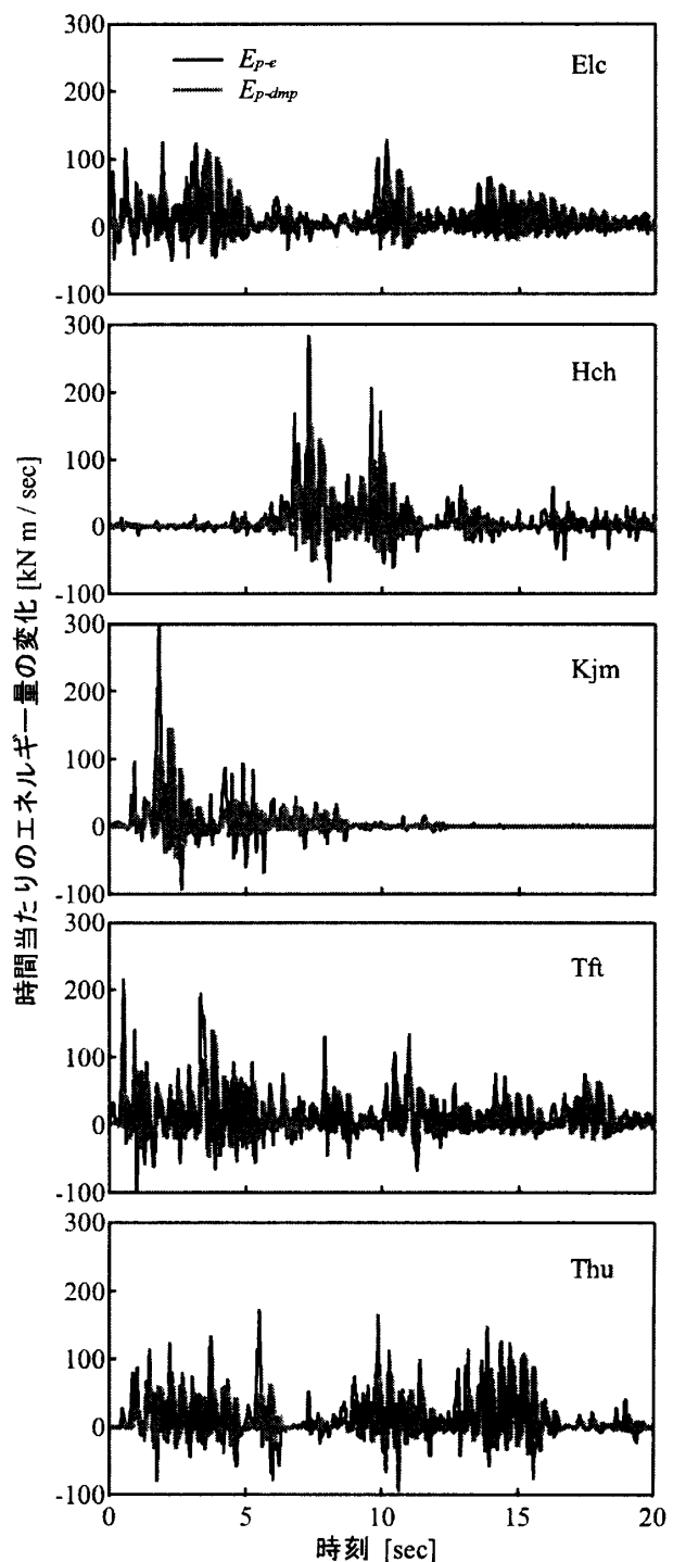
図-5 時間当たりのエネルギー量の変化
