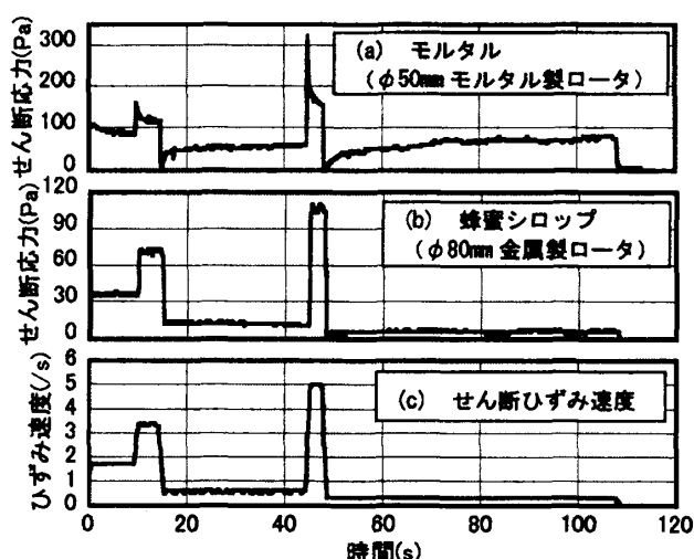
図-10 せん断応力およびせん断ひずみ速度の時刻歴
