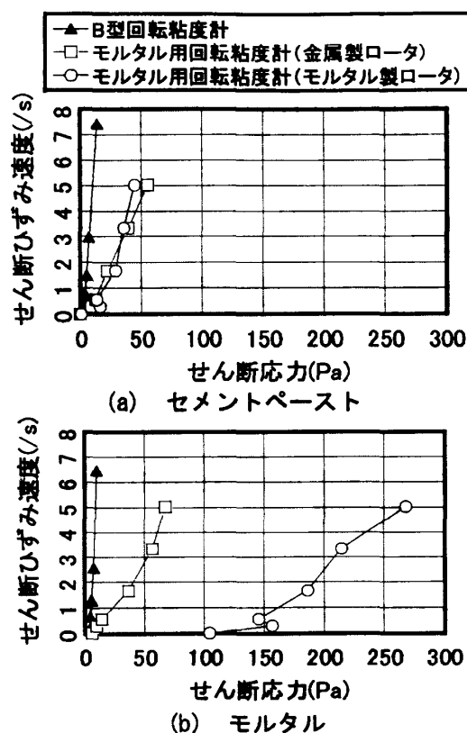
図-8 コンシステンシー曲線
