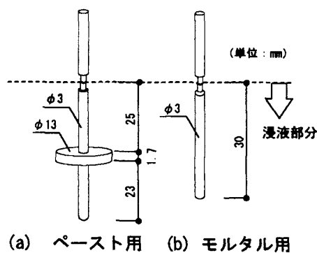
図-7 B型回転粘度計のロータ形状
