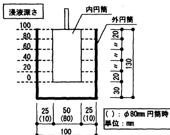
図-1 内円筒の浸液深さ
