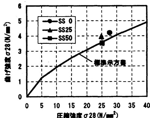
図-12 圧縮強度と曲げ強度の関係
