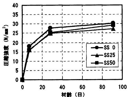
図-9 圧縮強度の発現状況
