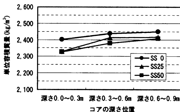
図-8 コアの深さ位置と単位容積質量
