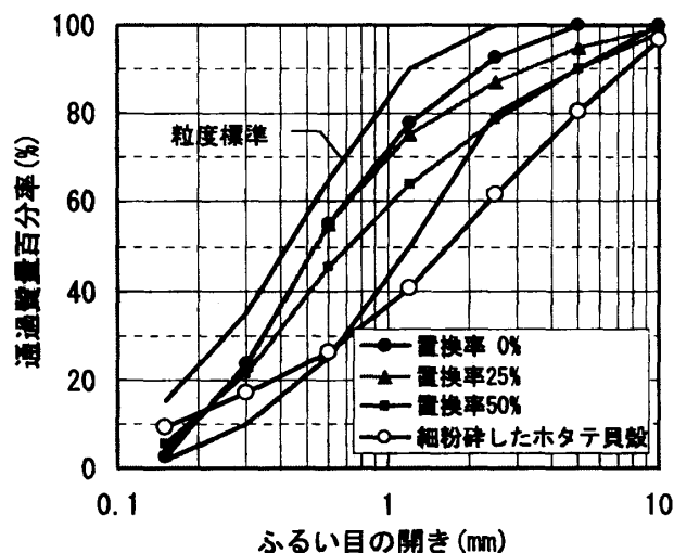
図-4 粒度分布
