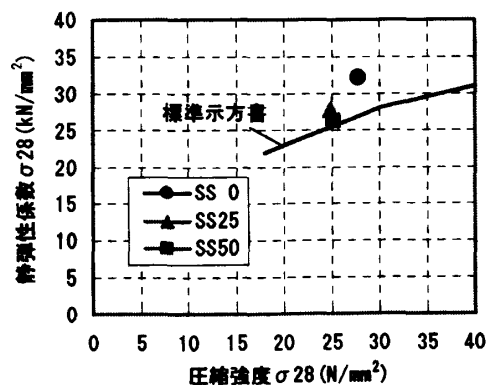
図-10 圧縮強度と静弾性係数の関係
