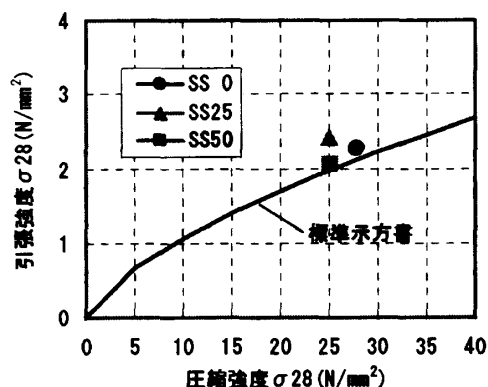
図-11 圧縮強度と引張強度の関係
