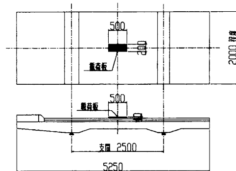
図-1 載荷方法
