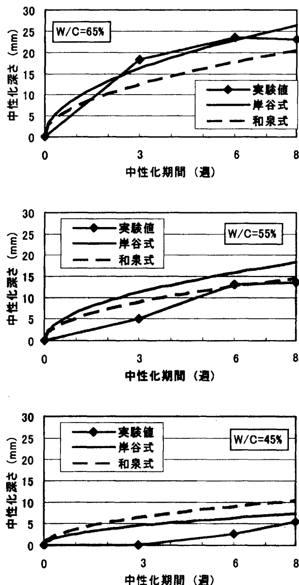
図-6 健全部での中性化促進期間と中性化深さの関係
