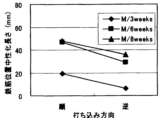
図-15 打ち込み方向と鉄筋位置中性化長さとの関係
