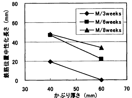
図-14 かぶり厚さと鉄筋位置中性化長さとの関係
