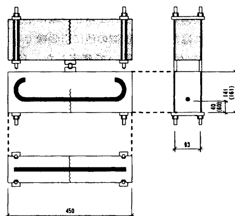
図-1 試験体図
