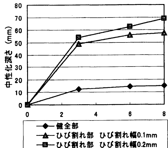
図-13 中性化促進期間と中性化深さの関係
