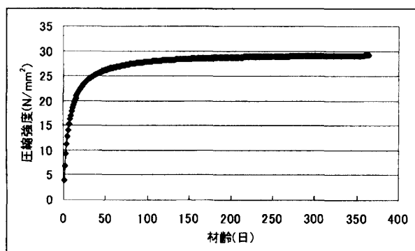
図-3 圧縮強度
