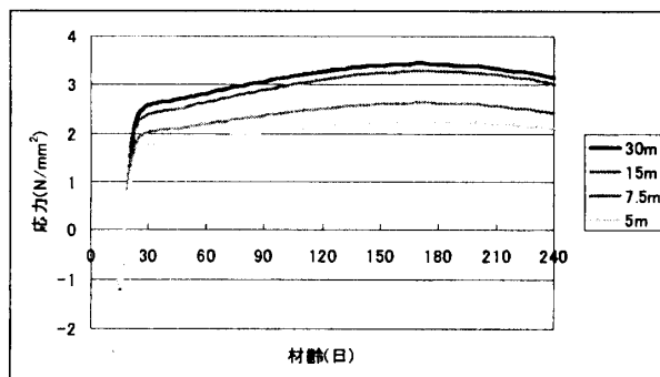
図-10 応力履歴
