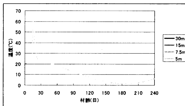
図-9 温度履歴
