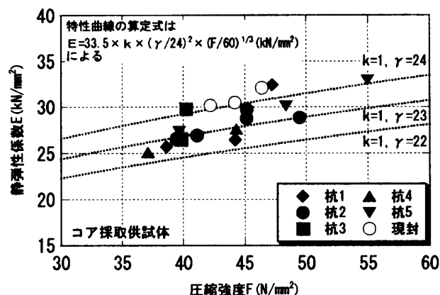
図-10 構造体コンクリートの静弾性係数
