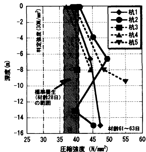
図-9 軀体強度分布
