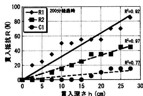
図-2 貫入抵抗
