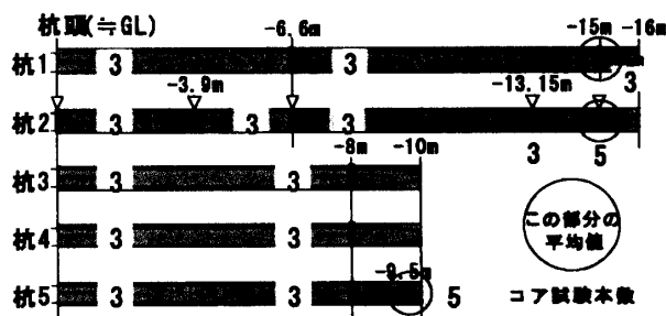
図-7 杭躯体コア採取位置及び本数
