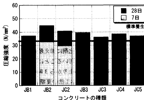
図-8 圧縮強度
