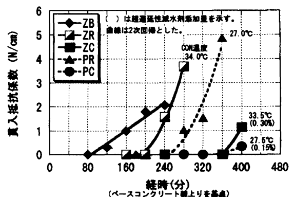
図-5 貫入抵抗係数と経過時間の関係
