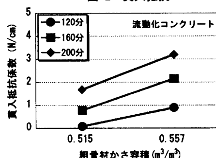
図-3 貫入抵抗係数と粗骨材かさ容積の関係
