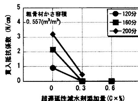
図-4 貫入抵抗係数と超遅延性減水剤添加量の関係
