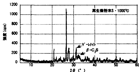
図-6 再生微粉末SのX線回折結果
