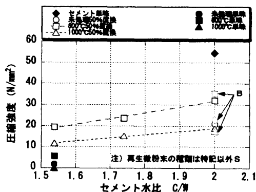
図-12 モルタルの圧縮強度
