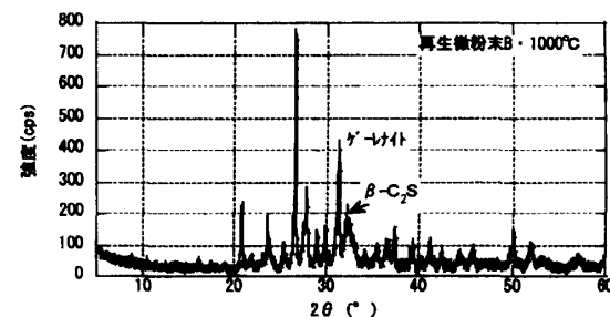
図-7 再生微粉末BのX線回折結果
