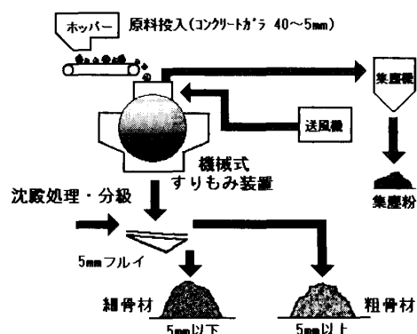
図-1 再生骨材の製造方法
