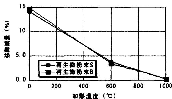
図-4 再生微粉末の強熱減量
