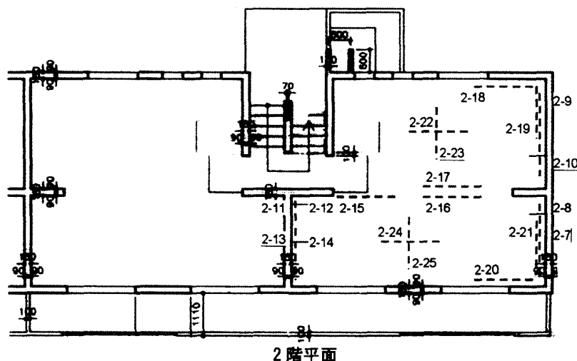
図-1 測線の例
