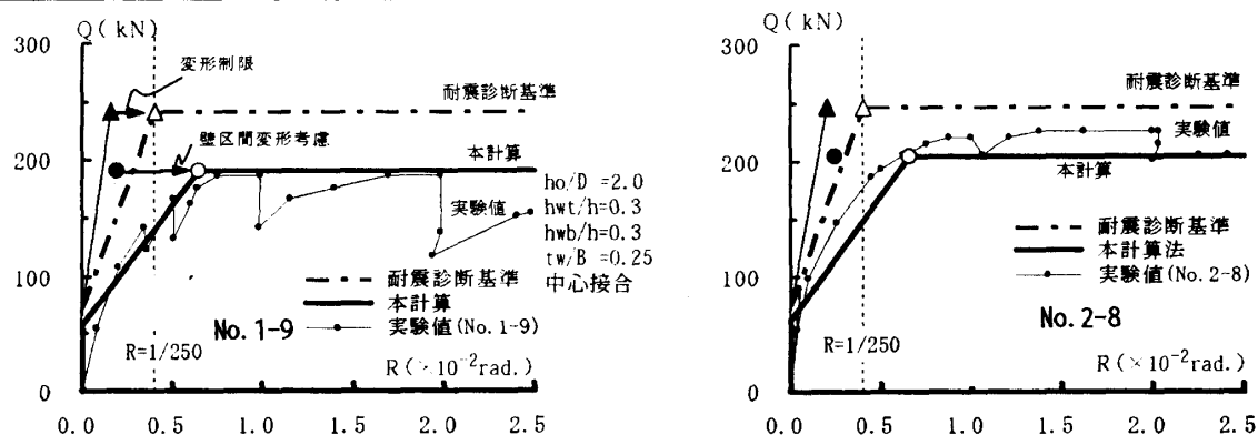
図-7 曲げ降伏した武田の試験体の荷重-変形角関係の実験結果 5) と計算結果の比較
