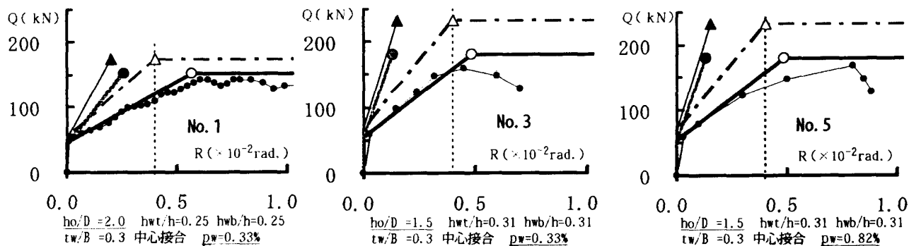
図-10 せん断破壊により耐力が決定した遠藤らの試験体の荷重-変形角関係の実験結果 13) と計算結果の比較
