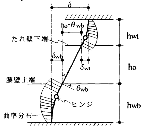
図-6 壁と接する区間の曲率による水平変形成分
