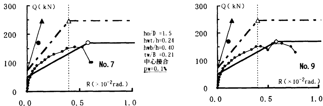
図-11 せん断破壊により耐力が決定した小室・広沢らの試験体の荷重-変形角関係の実験結果 14) と計算結果の比較
