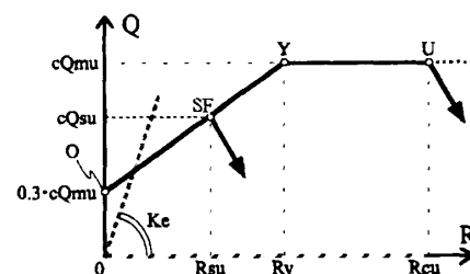
図－2 耐震診断基準での柱のせん断力－変形角関係
