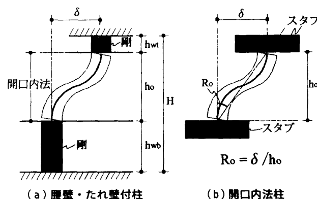
図－1 診断基準における腰壁・たれ壁付柱の扱い方
