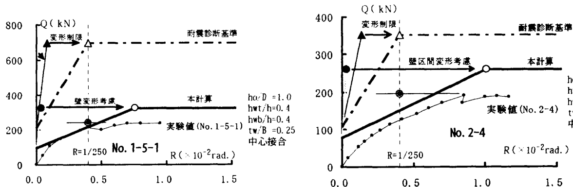
図-9 せん断破壊により耐力が決定した武田の試験体の荷重-変形角関係の実験結果 12) と計算結果の比較
