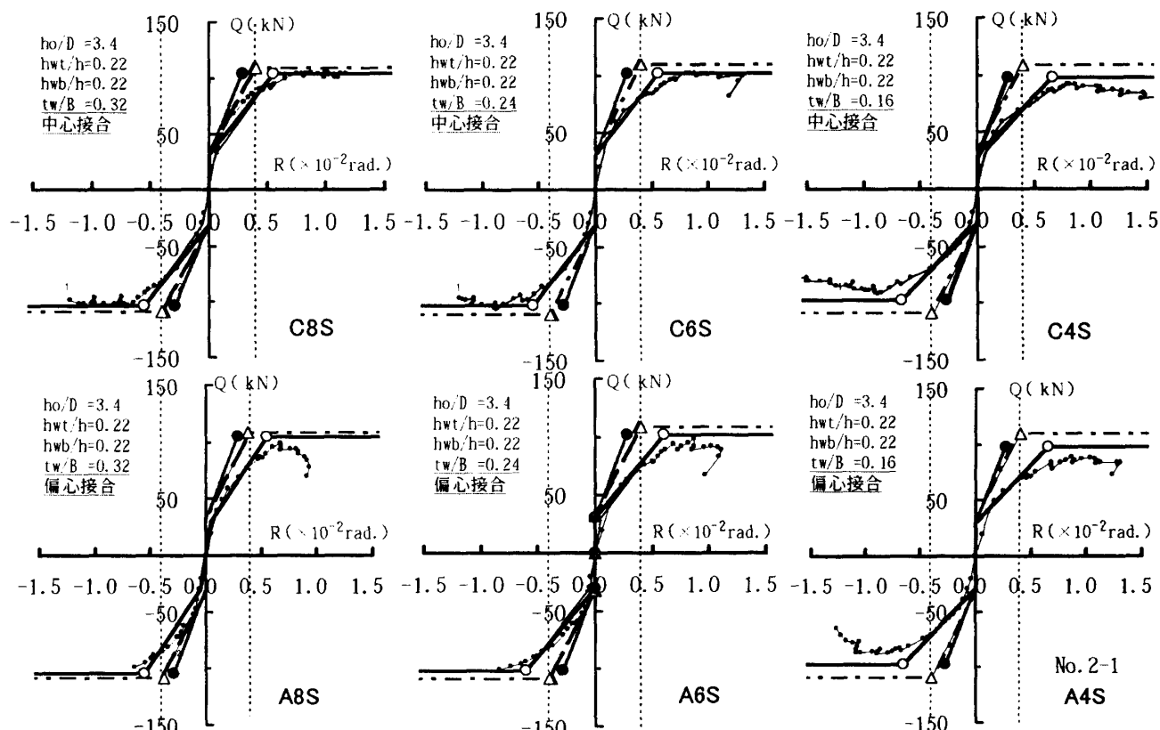
図-8 曲げ降伏した荒川の試験体の荷重-変形角関係の実験結果 6) と計算結果の比較
