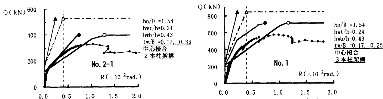
図-12 せん断破壊により耐力が決定した杉山らの試験体の荷重-変形角関係の実験結果 11)15) と計算結果の比較
