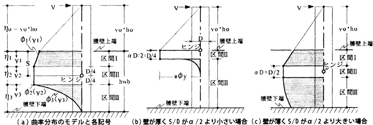
図-5 壁と接する区間の柱の曲率分布のモデルと記号
