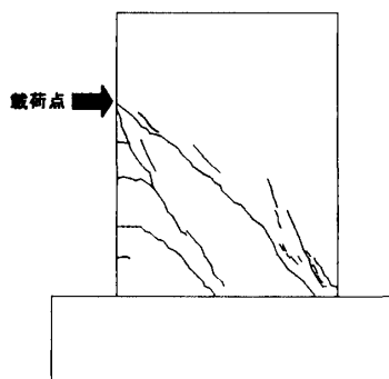
図-3 ひび割れ分布 No.13 (ひび割れが集中する場合)
