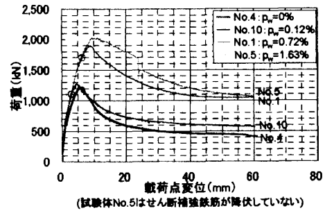
図-9 荷重変位関係 (パラメータ:せん断補強鉄筋比)
