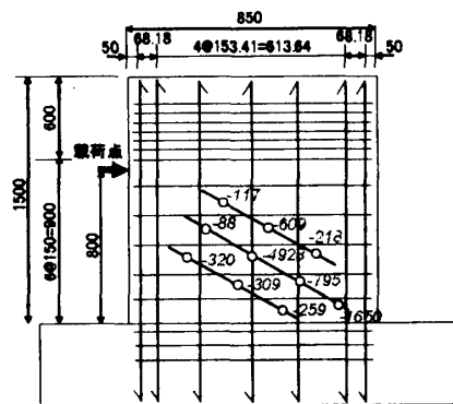
図-5 最大荷重時のコンクリート圧縮ひずみ (No. 10)
