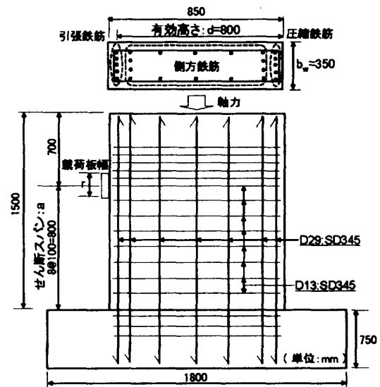
図-1 試験体の一例 (No.1)
