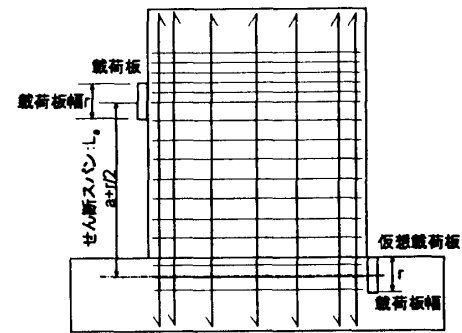
図-15 計算上のRC柱部材のせん断スパンの考え方
