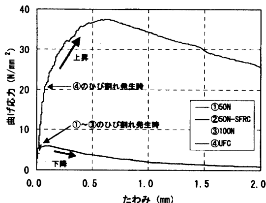
図-5 曲げタフネス試験結果
