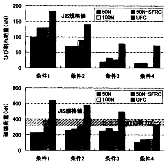
図－7 荷重条件ごとに 4 材料の比較
