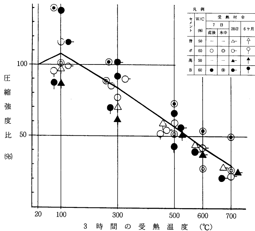
図一2 20℃の圧縮強度を100%とした場合の圧縮強度比と受熱温度との関係
