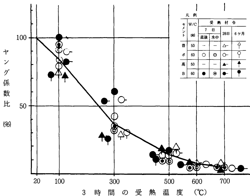
図-3 20℃のヤング係数を100%とした場合のヤング係数と受熱温度との関係
