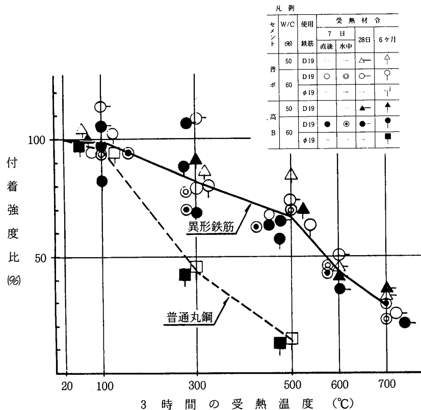
図一1 20°Cの付着強度を100%とした場合の付着強度比と受熱温度との関係
