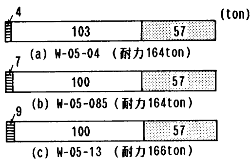
図-8 最下層での負担せん断力 (シアスパン比 0.5)
