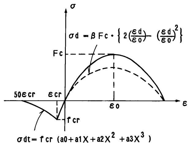
図-1 ひび割れ後の主応力-主ひずみ関係
