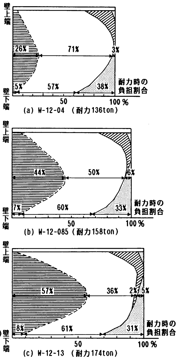
図-7 耐力時の負担せん断力の割合 (シアスパン比 1.2)
