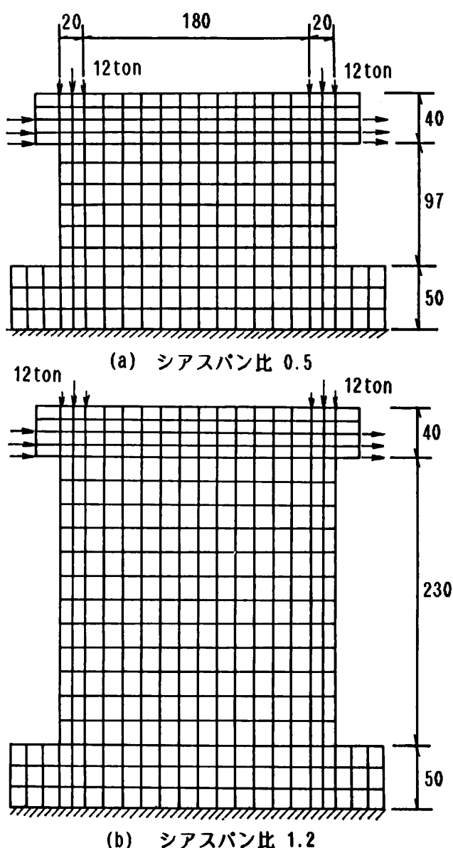
図-5 解析モデル (単位 cm)
