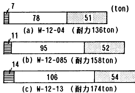
図-9 最下層での負担せん断力 (シアスパン比 1.2)
