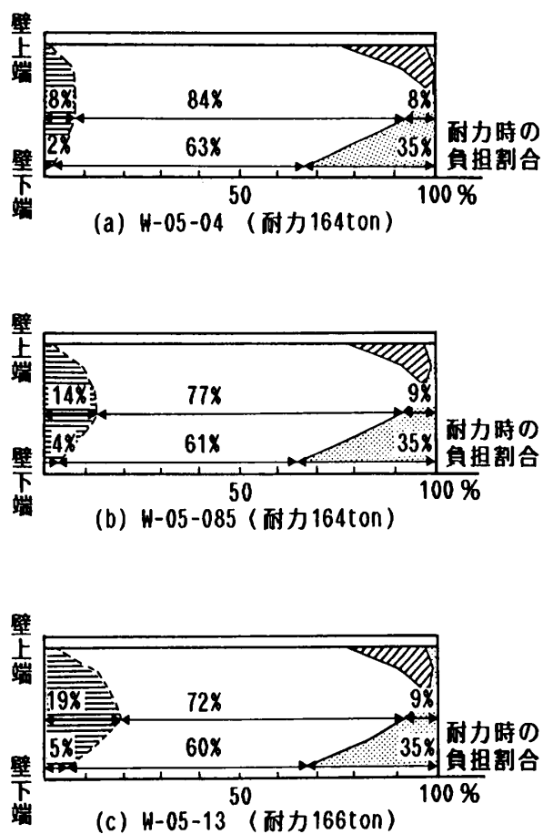
図-6 耐力時の負担せん断力の割合 (シアスパン比 0.5)
