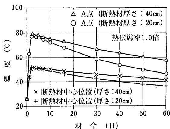
図-2 コンクリートおよび断熱材の温度履歴
