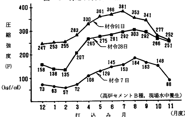
図-5 打込み月度と圧縮強度との関係
