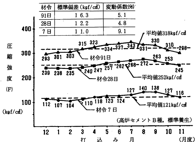
図-4 打込み月度と圧縮強度との関係
