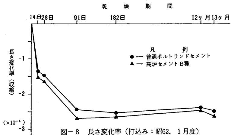
図-8 長さ変化率(打込み: 昭62. 1月度)
