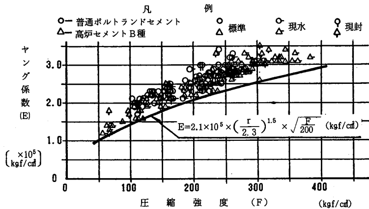
図-7 圧縮強度とヤング係数との関係
