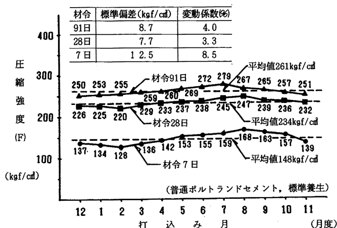
図-1 打込み月度と圧縮強度との関係
