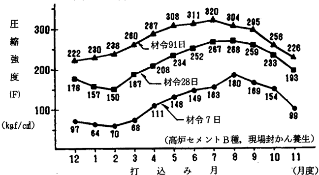
図-6 打込み月度と圧縮強度との関係
