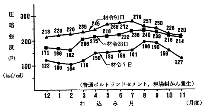
図-3 打込み月度と圧縮強度との関係
