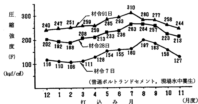
図-2 打込み月度と圧縮強度との関係
