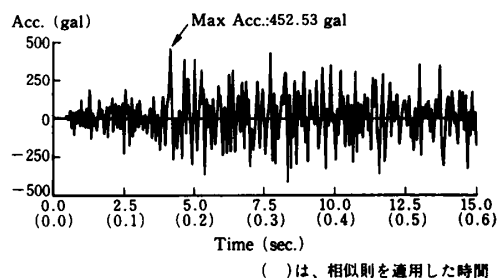
図-5 入力地震波
