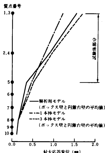
図-6 最大応答変位の比較
