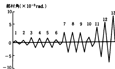
図-8 加力スケジュール
