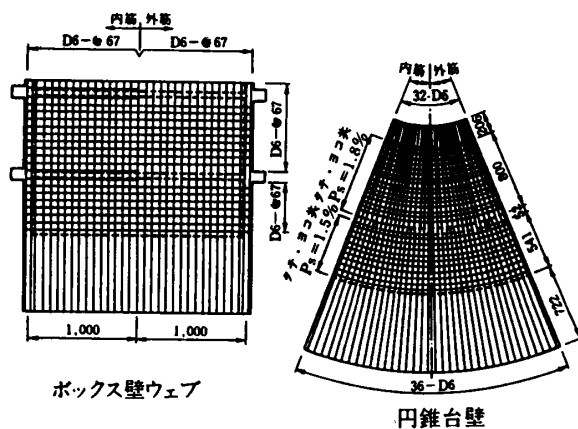
図-2 配筋図
