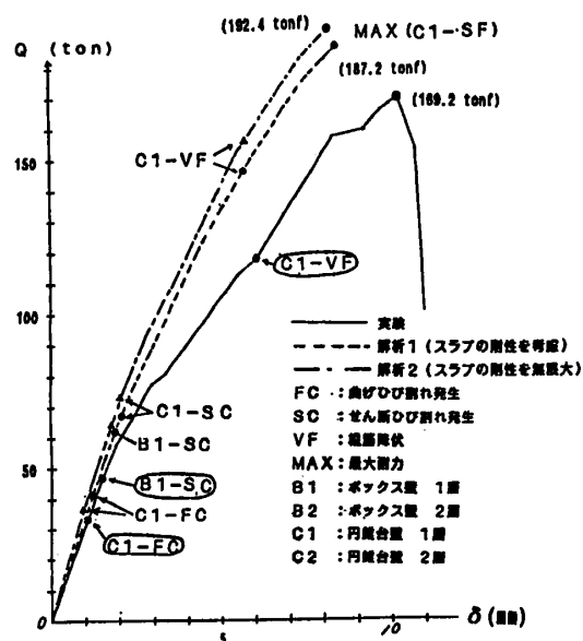
図-16 荷重-全体変形関係
