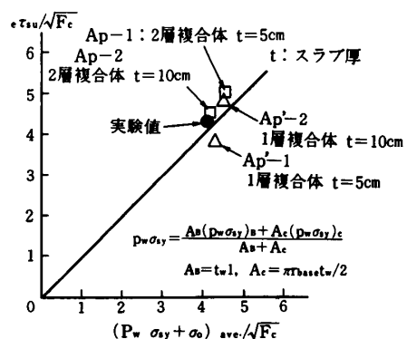
図-13 最大耐力の実験と計算値の比較
