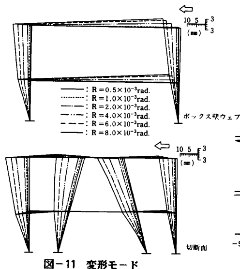
図-11 変形モード
