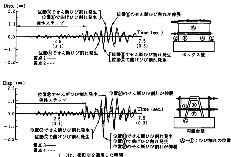
図-7 変位時刻歴
