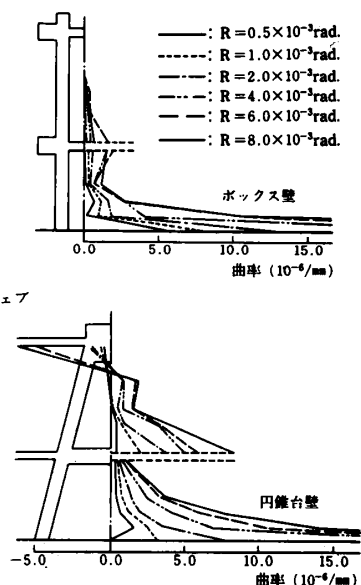
図-12 曲率分布
