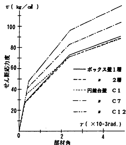
図-15 せん断変形包絡線
