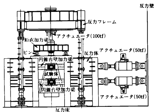
図-3 加力装置の概要
