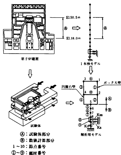
図-4 建屋のモデル化
