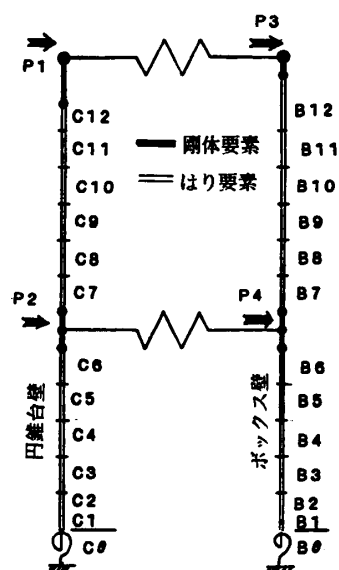
図-14 解析モデル
