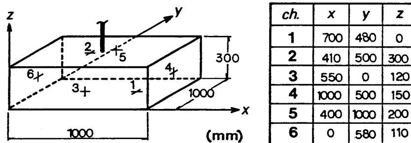
図-1. 供試体寸法およびセンサー位置
