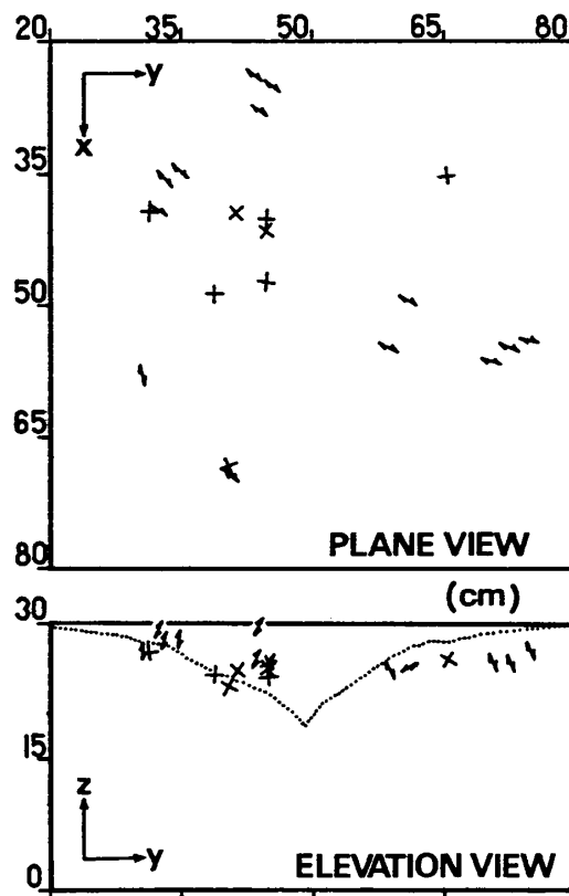
図-7(D). AE源位置および逆解析結果(第4段階) ( \leftrightarrow 引張卓越型, \times せん断卓越型)
