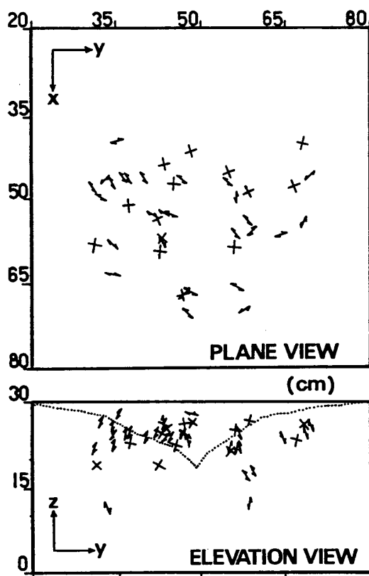
図-7(C). AE源位置および逆解析結果(第3段階) ( \leftrightarrow 引張卓越型, \times せん断卓越型)
