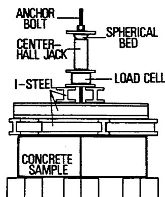
図-4.載荷装置
