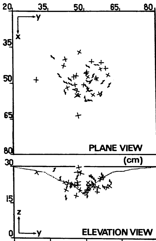
図-7A. AE 源位置および逆解析結果 (第1段階) ( \rightarrow 引張卓越型, \times せん断卓越型)
