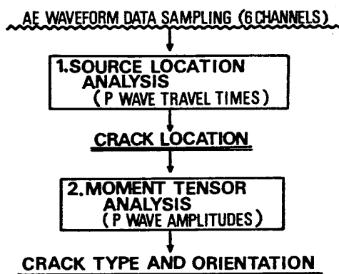
図-5. 逆解析フローチャート
