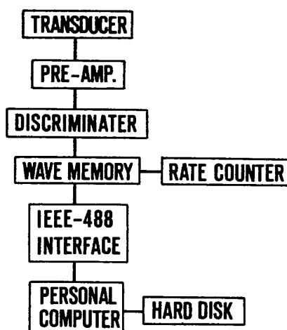
図-3.AE計測システム
