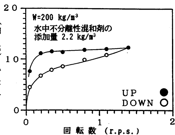
図-3 水中不分離性混和剤Aを用いたコンクリートのヒステリシスループ
