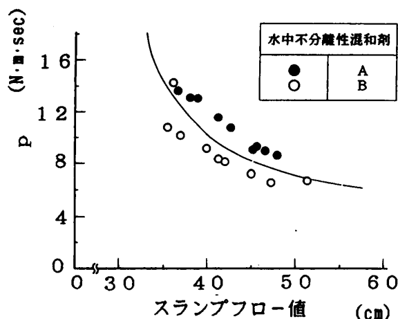
図-6 スランプフロー値とpの関係
