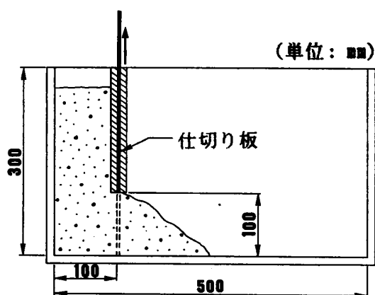
図-2 ボックスフロー試験装置
