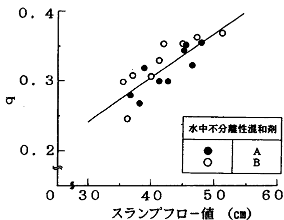
図-7 スランプフロー値とqの関係
