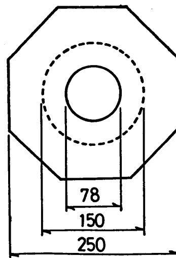
図-3 . 八角柱供試体
