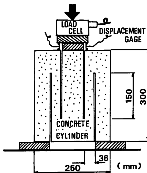
図-4 . 試験装置
