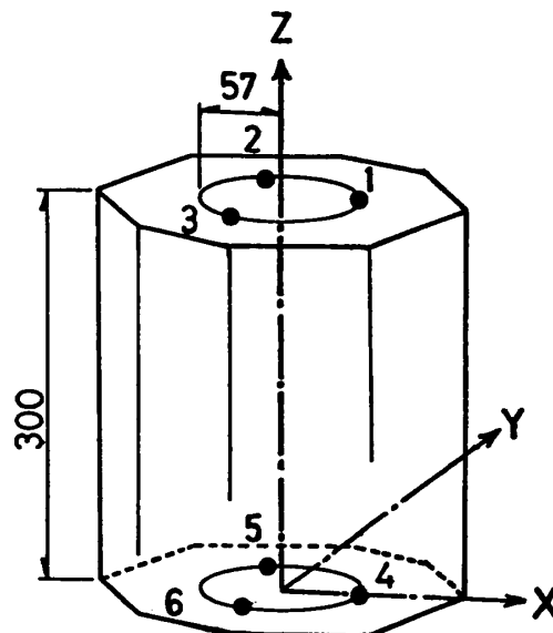
図－7. トランスデューサー配置
