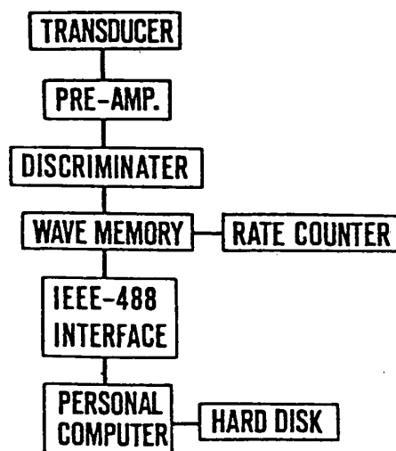
図－6. A E計測装置
