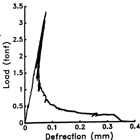
図-5 . 荷重 - 変位
