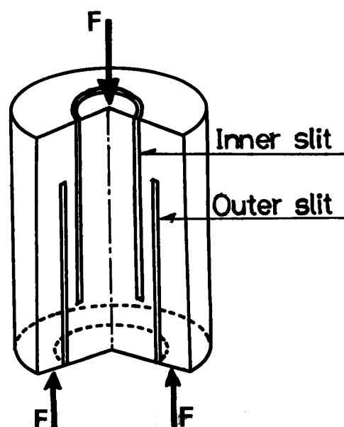
図-2. 円筒引張試験
