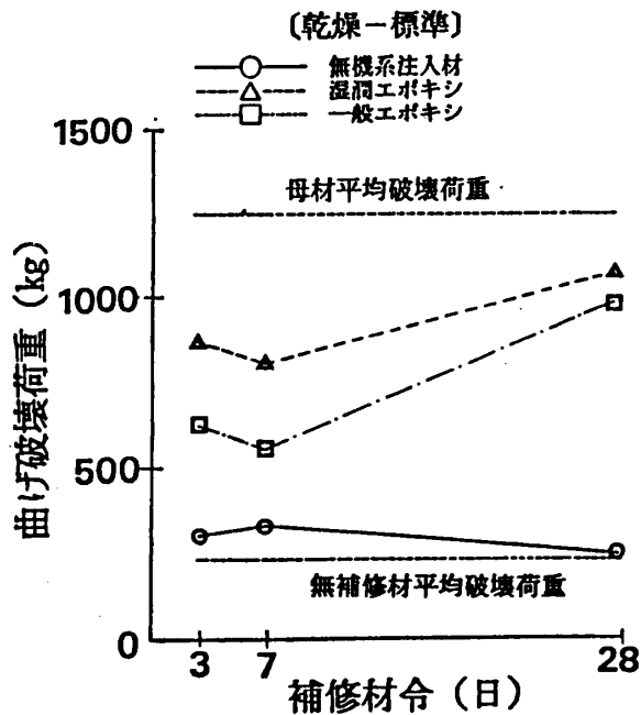
図-6 材令～曲げ破壊荷重(シリーズ 3)
