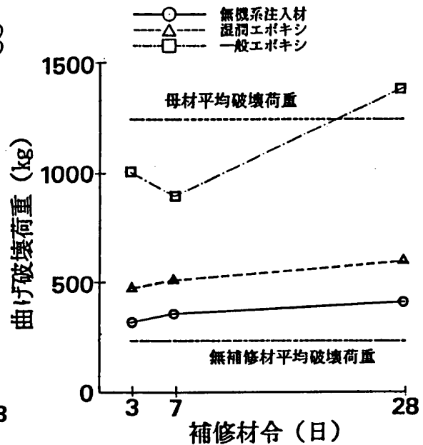
図-5 材令～曲げ破壊荷重(シリーズ 2)
