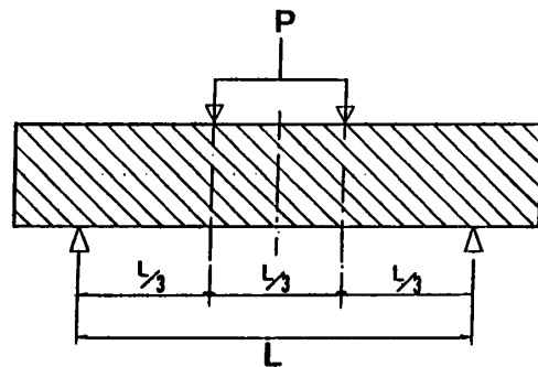
図-2 曲げ破壊試験
