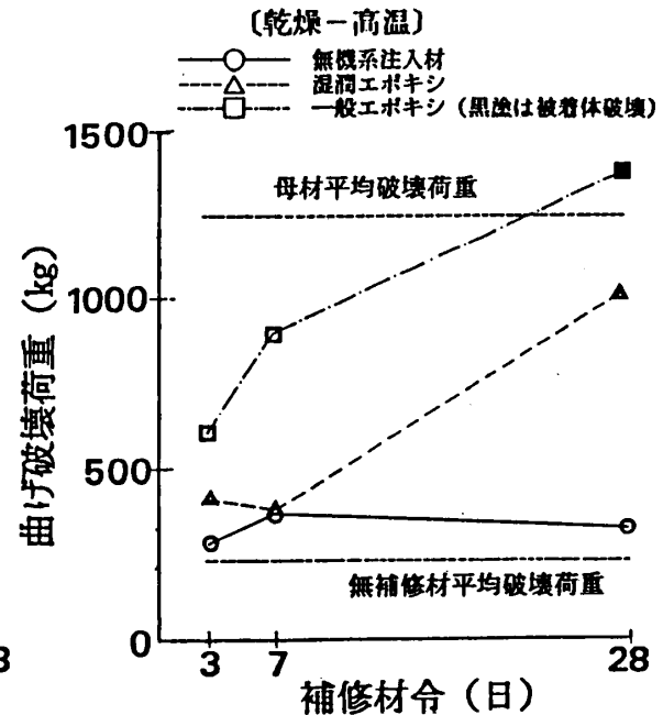
図-7 材令～曲げ破壊荷重(シリーズ 4)
