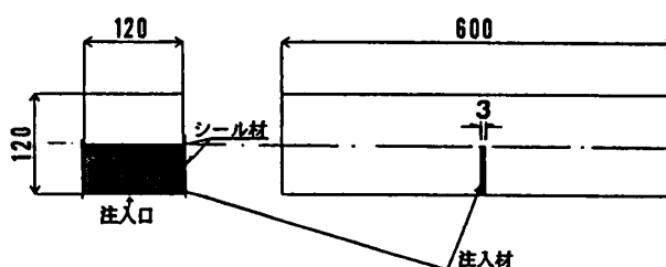
図-1 実験供試体寸法・形状
