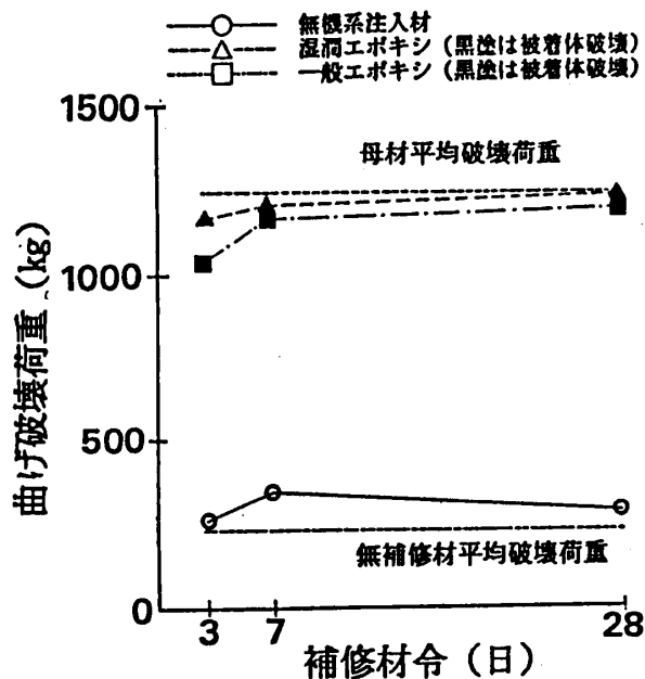
図-4 材令～曲げ破壊荷重(シリーズ 1)
