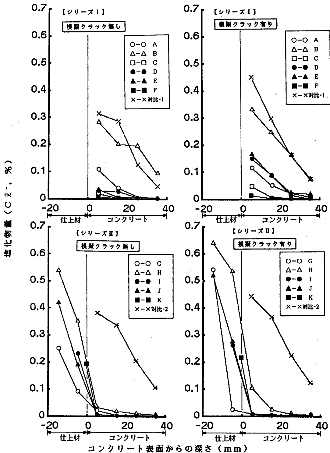
図-3 塩化物の分布図
