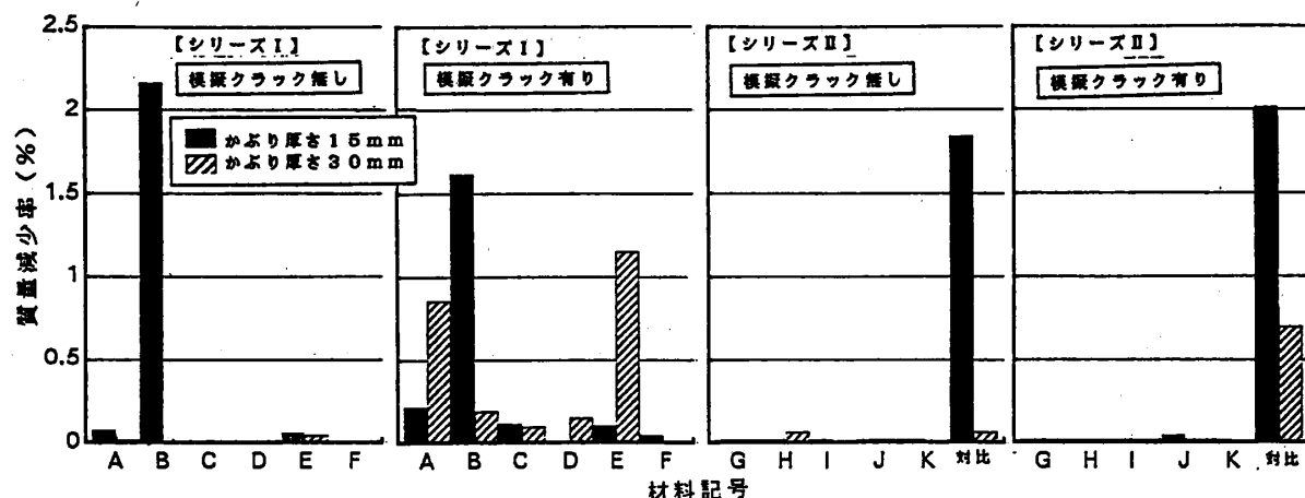
図-6 材料別の質量減少率
