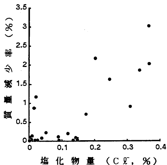
図-5 質量減少率と 塩化物量の関係
