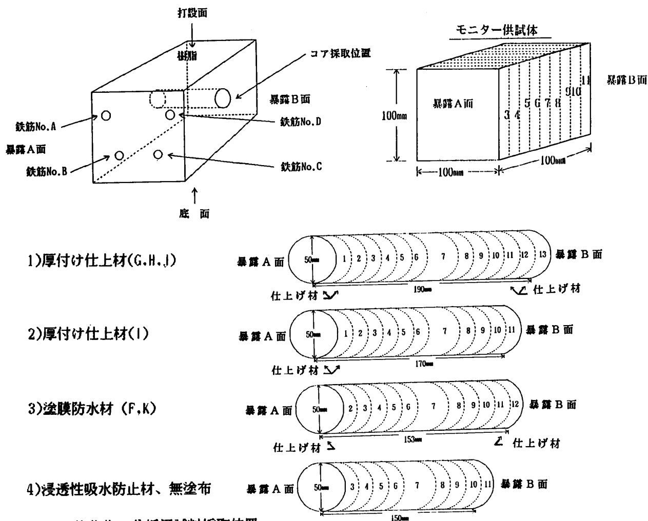
図-2 塩化物の分析用試料採取位置
