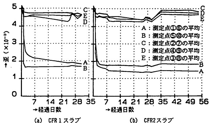
図10 PC鋼線の経時歪（プレストレス導入時～載荷直前）
