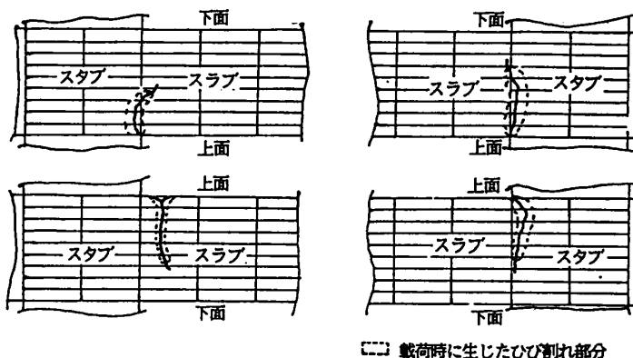
図8 CFR2スラブの端部ひび割れ図
