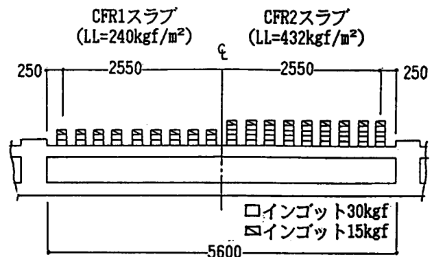
図3 持続載荷時載荷状態（18点集中載荷）
