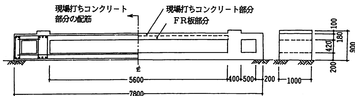
図1 試験体形状図 (単位: mm)
