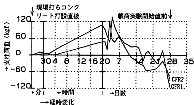
図7 支柱荷重の経時変化
