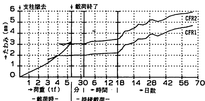
図9 スラブ下面中央のたわみ
