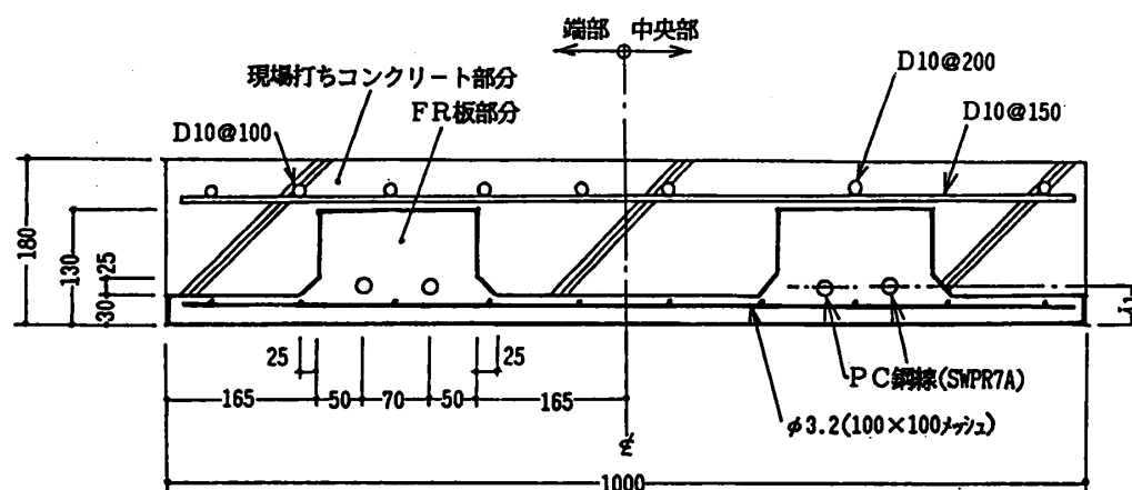
図2 断面詳細図 (単位: mm)
