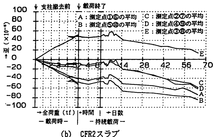
図11 PC鋼線の経時歪（載荷時支柱撤去前基準）
