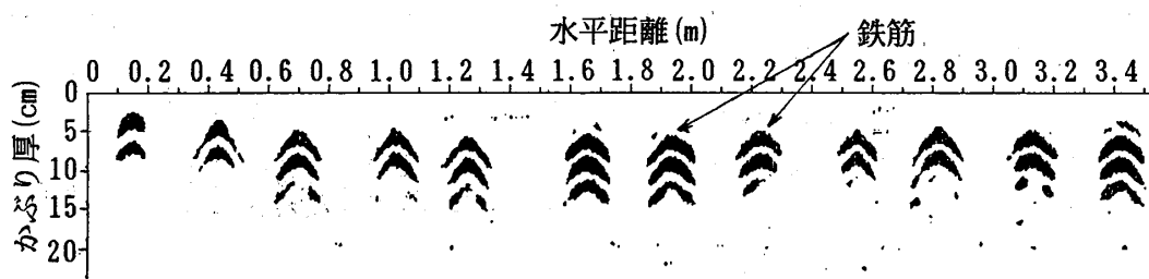
図-2 レーダー法による鉄筋ピッチおよびかぶり厚さの測定結果(導流壁)
