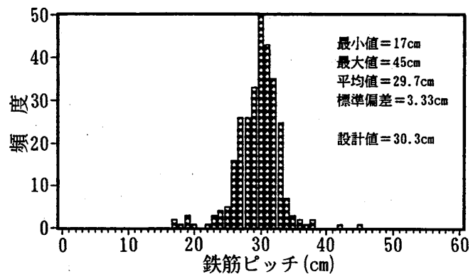
図-4 鉄筋ピッチの統計量(導流壁)
