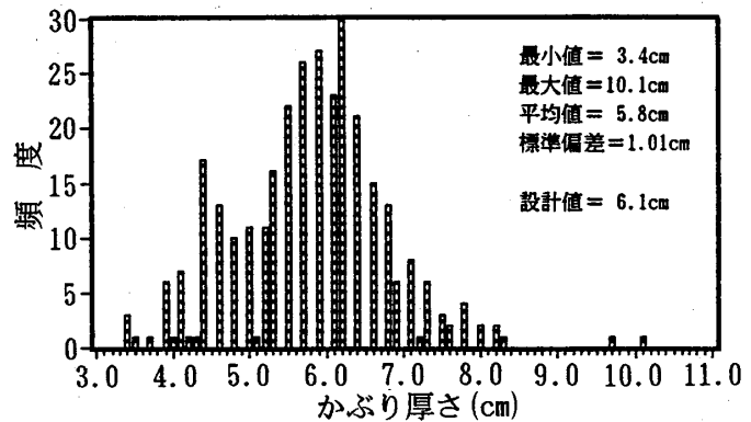
図-3 かぶり厚さの統計量(導流壁)
