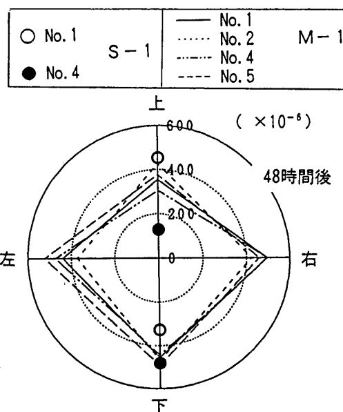
図-6 定着体1における鋼管円周方向のひずみ分布 (S-1, M-1)
