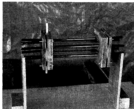
写真-1 実物モデル注入試験装置
