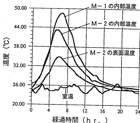
図-12 定着体 2 における温度変化
