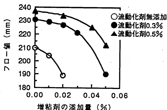
図-4 増粘剤および流動化剤添加量とフロー値との関係
