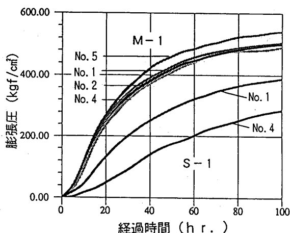
図-9 定着体1における膨張圧経時変化 (S-1, M-1)
