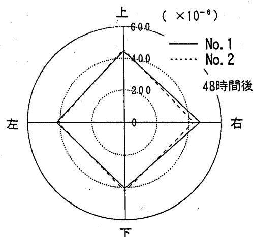
図-8 垂直方向充填の場合の鋼管円周方向のひずみ分布 (S-1)
