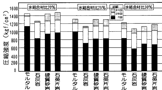
図-2 標準養生試験体の圧縮強度
