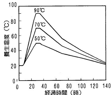
図-1 初期高温養生の温度履歴
