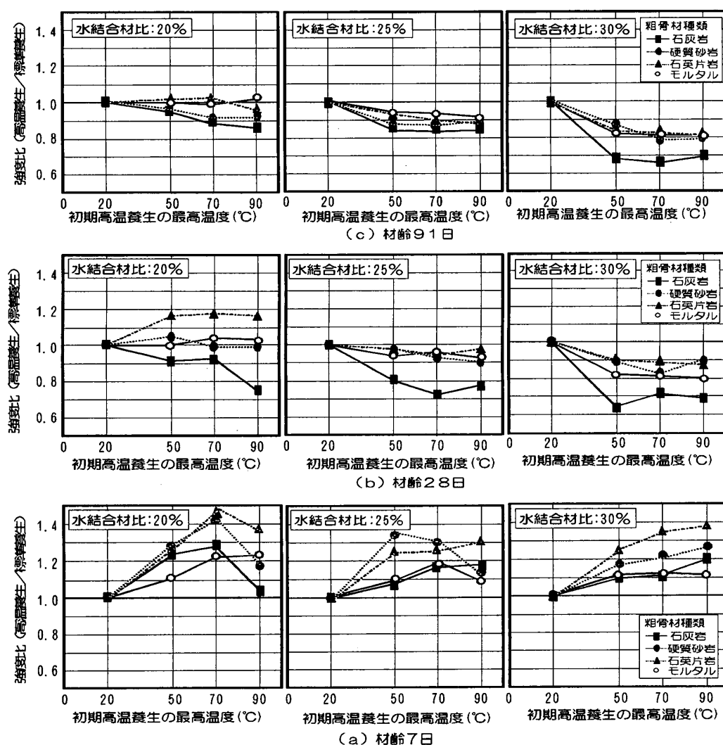
図-4 初期高温養生と標準養生の強度比
