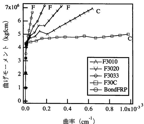
図-6 曲げモーメント-曲率関係 (L=30m)
