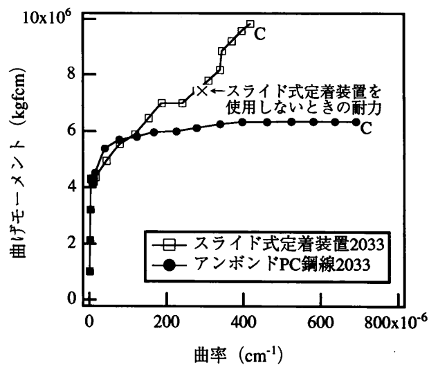
図-10 曲げモーメント-曲率関係
