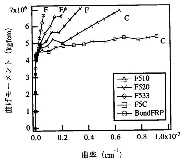
図-4 曲げモーメント-曲率関係（L=50m）
