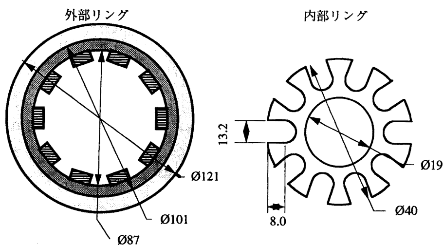
図-8 平面図
