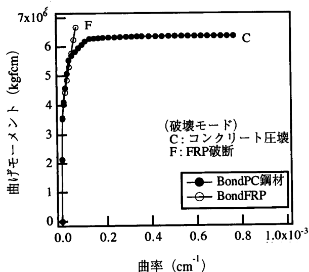
図-2 曲げモーメント-曲率関係（ボンド部材）
