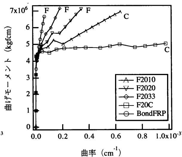
図-3 曲げモーメント-曲率関係（L=20m）
