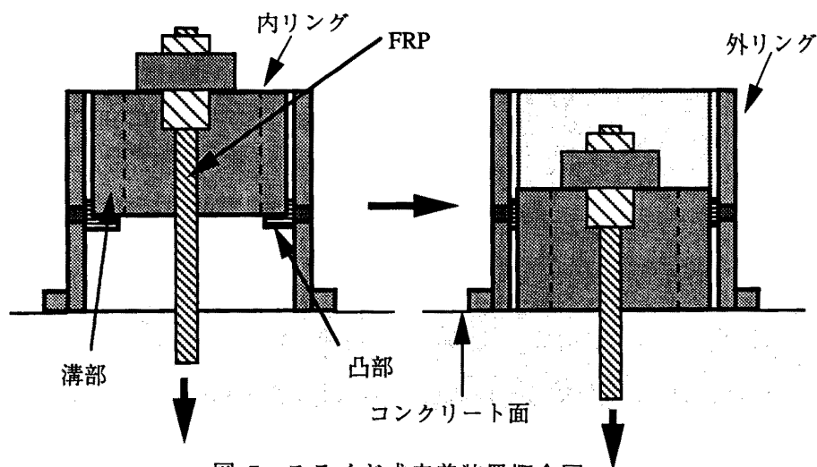
図-7 スライド式定着装置概念図
