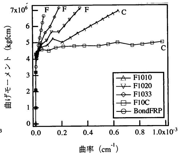
図-5 曲げモーメント-曲率関係（L=10m）
