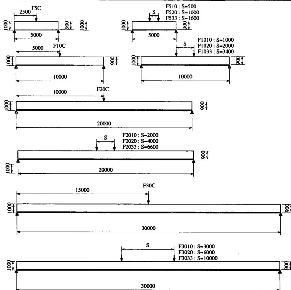
図-1 供試体の形状と载荷スパン (単位: mm)
