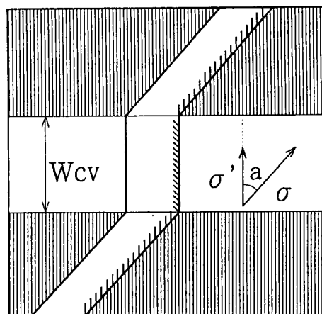
図－7 らせん鉄筋による拘束の概念
