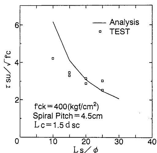
図－8 重ね長さとは終局荷重の関係
