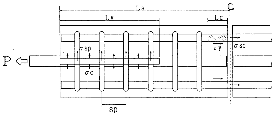
図-1 仮定破壊モード(1)
