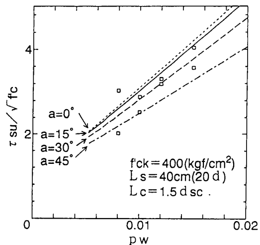
図-6 横補強筋量と終局強度の関係
