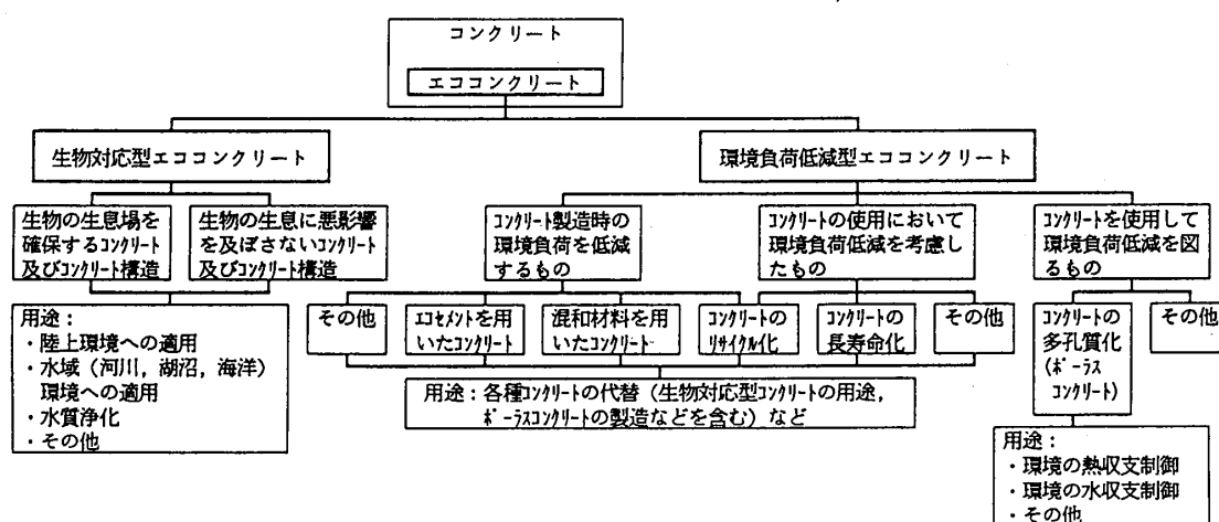
図3 エココンクリートの分類と用途
