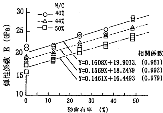
図3-A 弾性係数と砂含有率（実験A）
