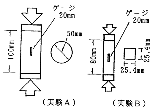
図 1 圧 縮 試 験
