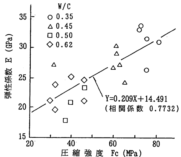
図4-A 弾性係数 (E) と圧縮強度 (Fc) -実験A- 図4-B 弾性係数 (E) と圧縮強度 (Fc) -実験B-
