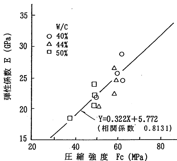
図4-A 弾性係数 (E) と圧縮強度 (Fc) -実験A- 図4-B 弾性係数 (E) と圧縮強度 (Fc) -実験B-
