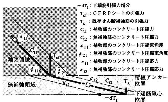
図ー4 U字巻・梁側面アンカー試験体における力の釣合いの仮定
