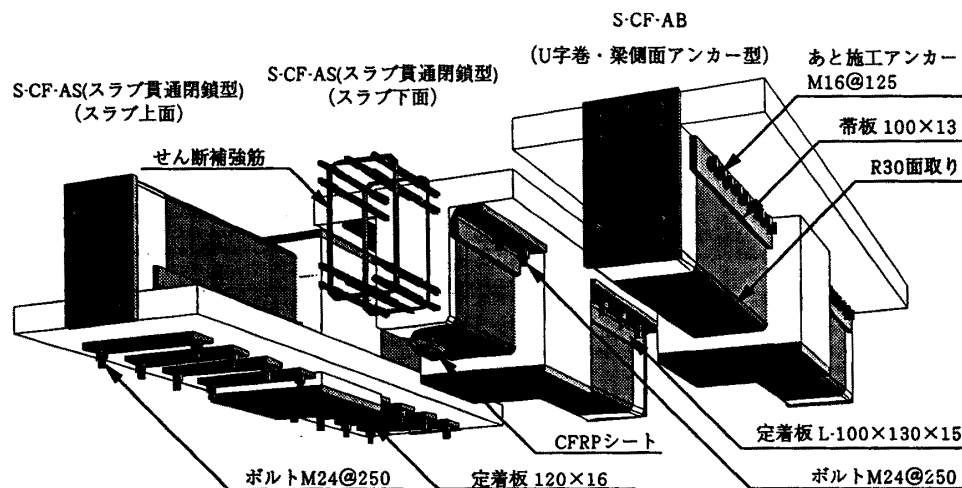
図-2 CFRP シートのアンカー方法
