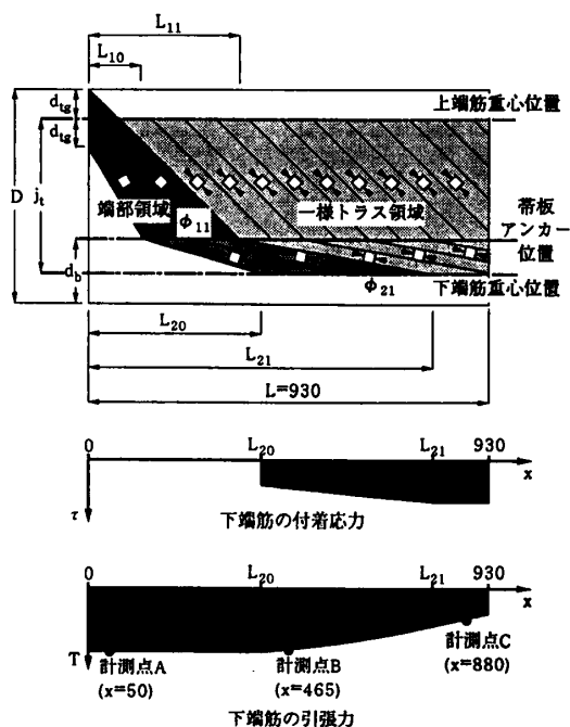
図-5 U字巻・梁側面アンカー試験体のトラス作用応力状態の仮定
