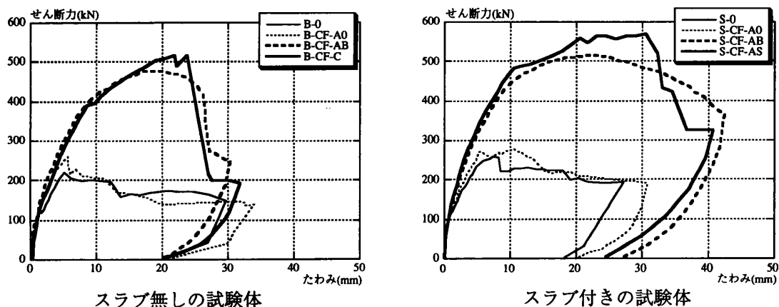
図ー3 せん断力～変位関係
