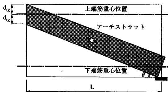
図-6 アーチ作用応力状態
