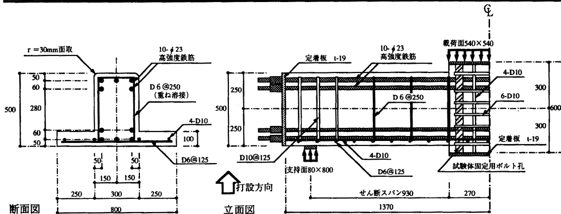
図-1 試験体の配筋と荷重条件
