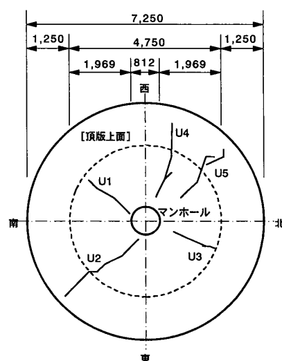
図-6 施工後の頂版のひび割れ分布
