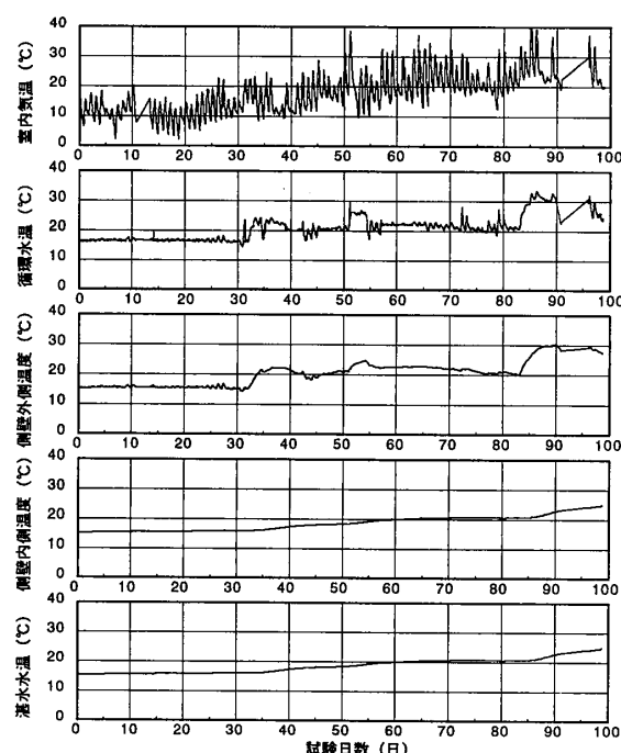
図-7 長期透水試験中の温度経時変化
