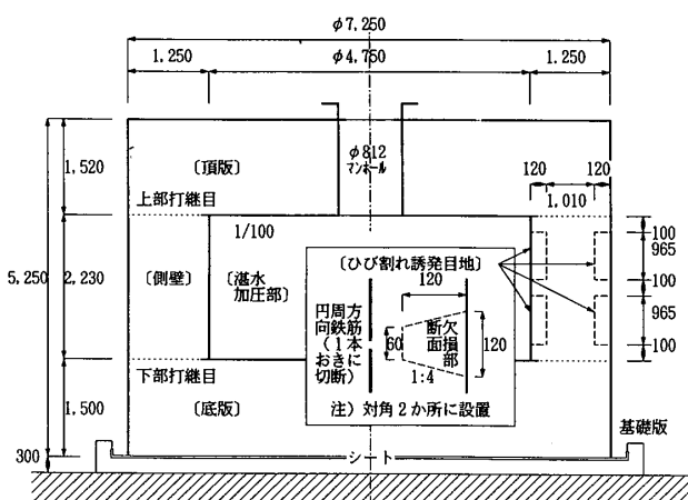
図-2 ひび割れ誘発試験体の構造概要
