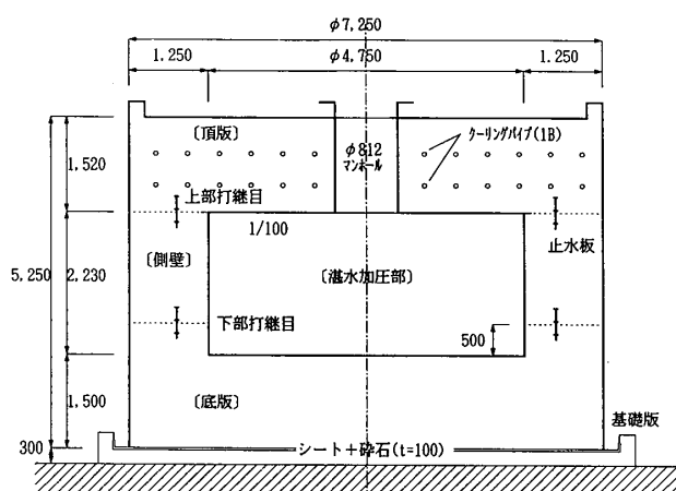
図-1 ひび割れ制御試験体の構造概要
