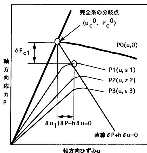
図-2 初期不整と応力ひずみ曲線
