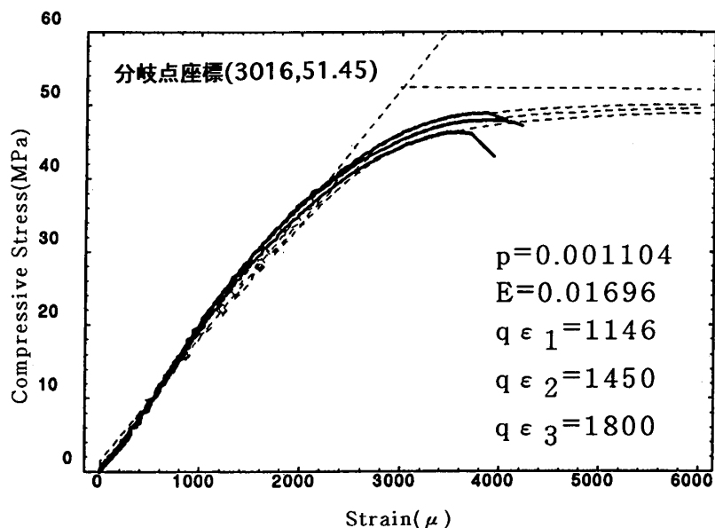
図-6 シミュレーションの例(分岐)
