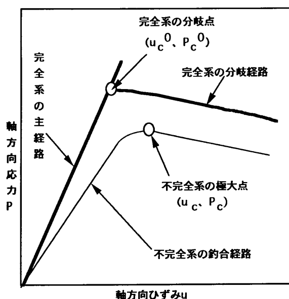
図-1 分岐現象の例
