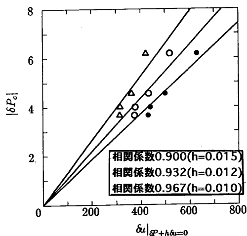
図-5 初期不整感度則の適合性(分岐)
