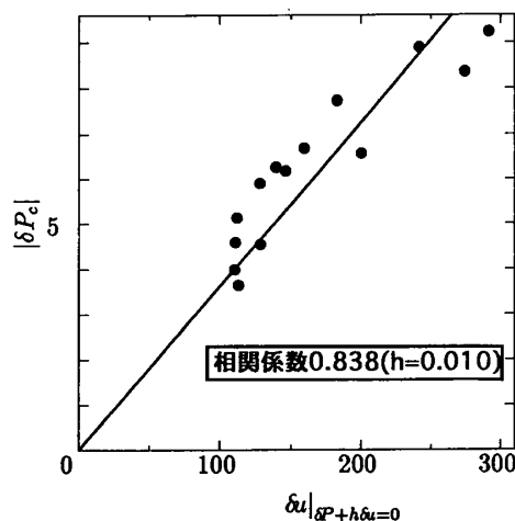
図-4 初期不整感度則の適合性(全体)
