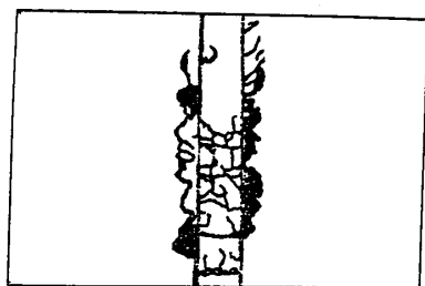
図-12 ひび割れ図(LJ20-15)
