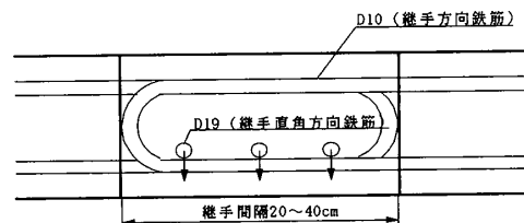
図-5 ループ継手の詳細図
