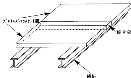
図－1 継手を有する床版の例
