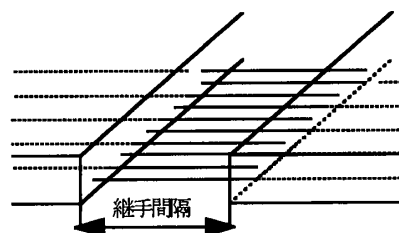
図－2 ラップ継手構造
