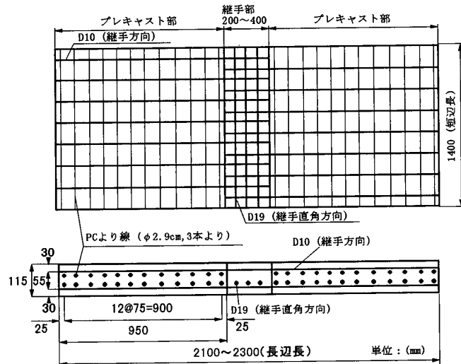
図-4 供試体の概要
