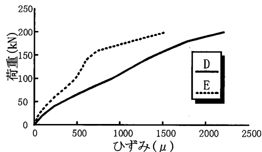
図－9 継手方向鉄筋の荷重－ひずみ曲線
