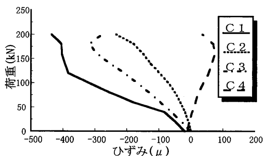
図－10 荷重－圧縮側コンクリートひずみ関係
