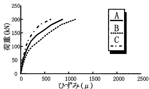
図－7 継手直角方向鉄筋の荷重－ひずみ曲線
