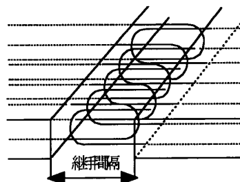
図－3 ループ継手構造
