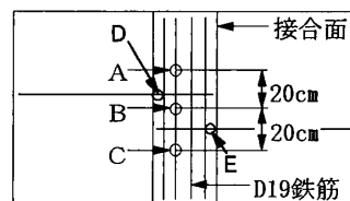
図－8 ひずみゲージの貼付位置
