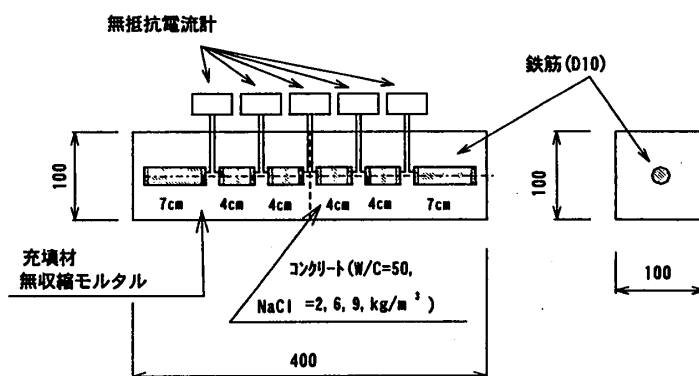
図-3 マクロセル電流測定用供試体
