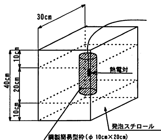
図-2 水和熱測定試験装置(簡易断熱)
