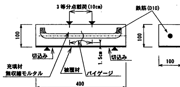
図-4 ひび割れ追従性試験用供試体
