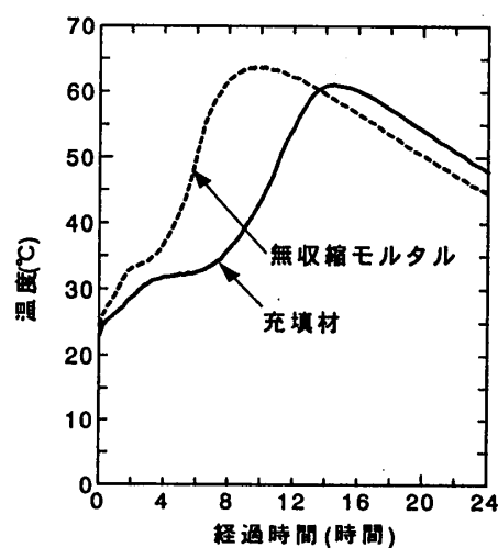
図-9 水和熱による温度上昇
