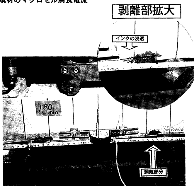
図-12 ひび割れ追従性
