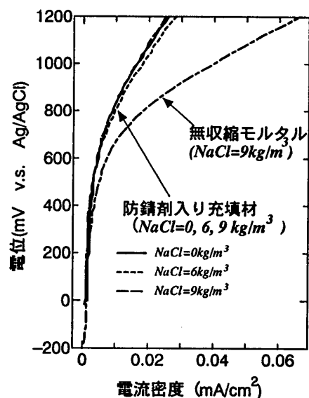
図-10 アノード分極曲線
