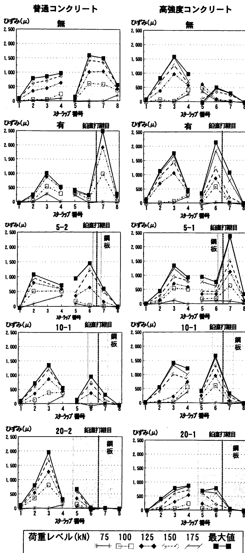
図-6 各荷重レベルにおけるスーラップのひずみ
