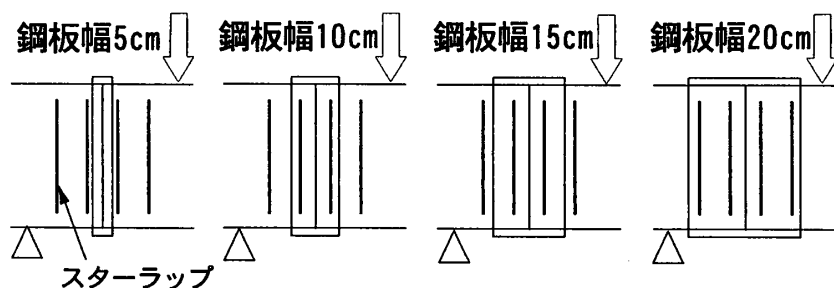
図-5 鋼板幅とスターラップの位置
