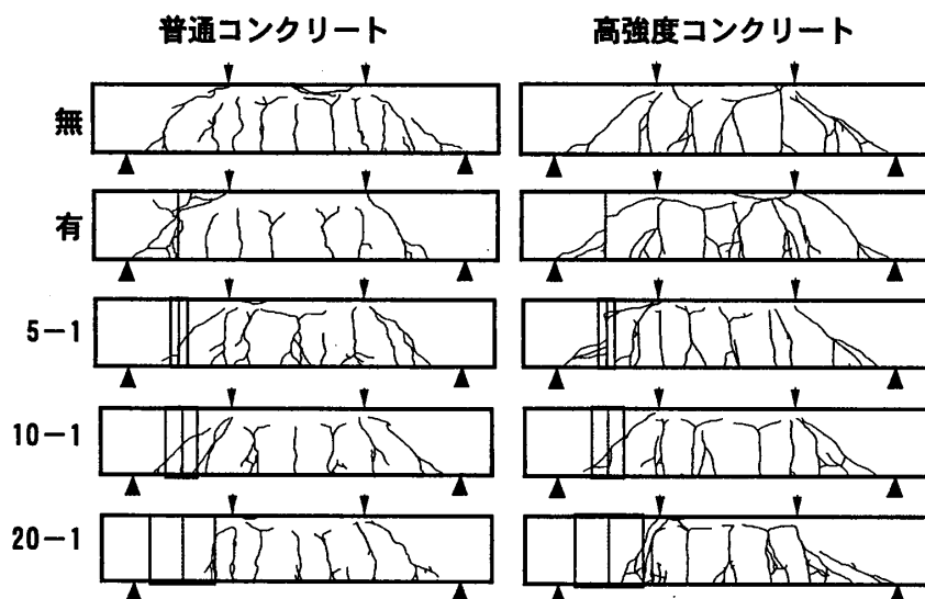
図-4 ひび割れの発生状況
