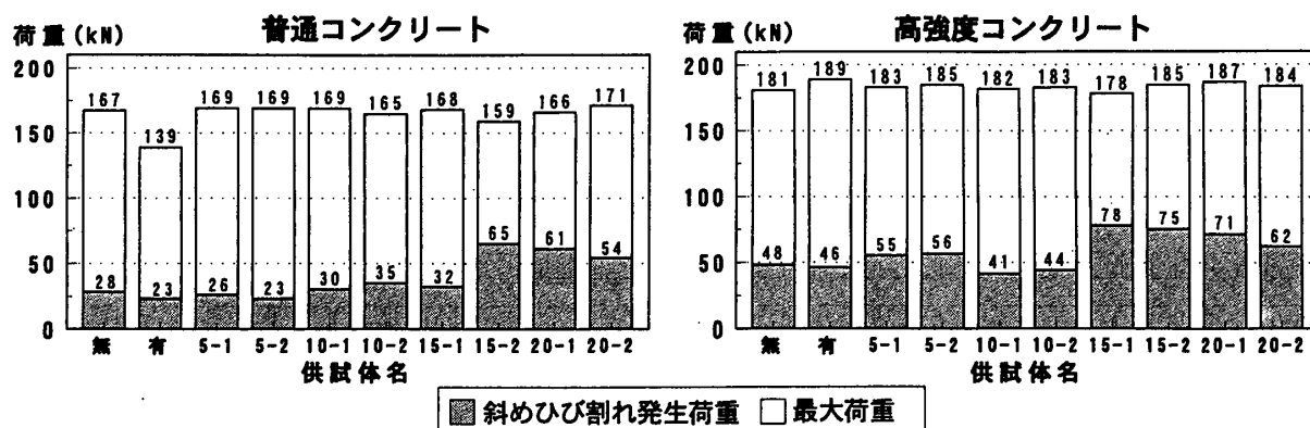
図-3 斜めひび割れ発生荷重および最大荷重
