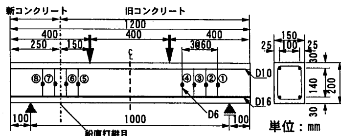
図-1 はり供試体の形状寸法
