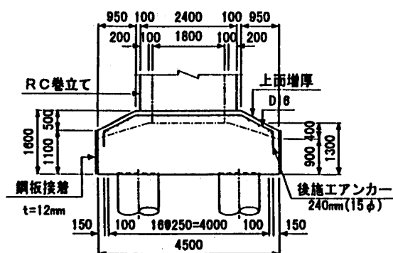
(a) 断面図
