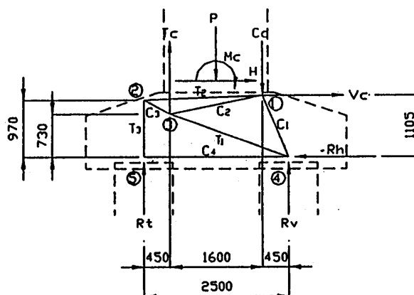
図-8 Strut-and-Tie モデル
