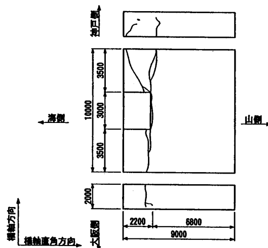
図-5 ひびわれ状況図②
