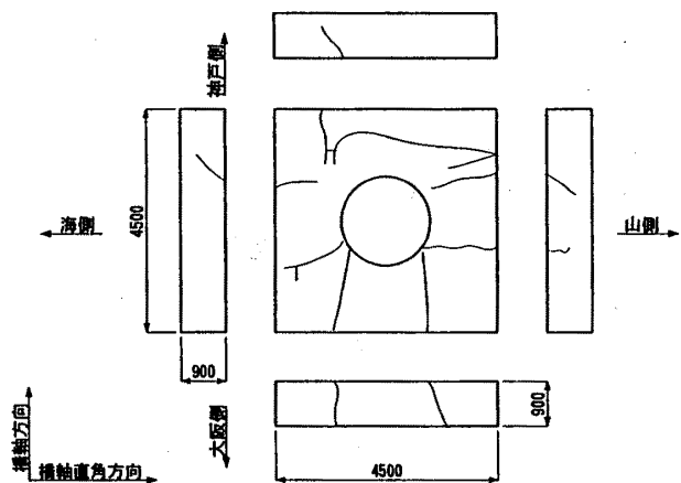
図-2 ひびわれ状況図①
