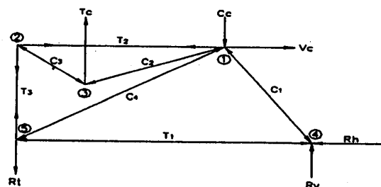
(b) ひびわれが発生する場合
