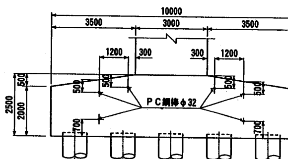
(a) 断面図
