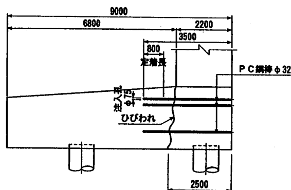
(b) 側面図
