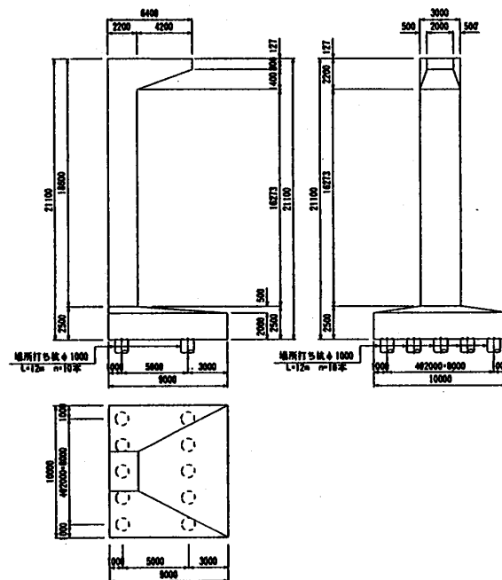
図-4 橋脚形状寸法図②
