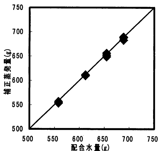
図-2 配合水量と補正蒸発量(ペースト)
