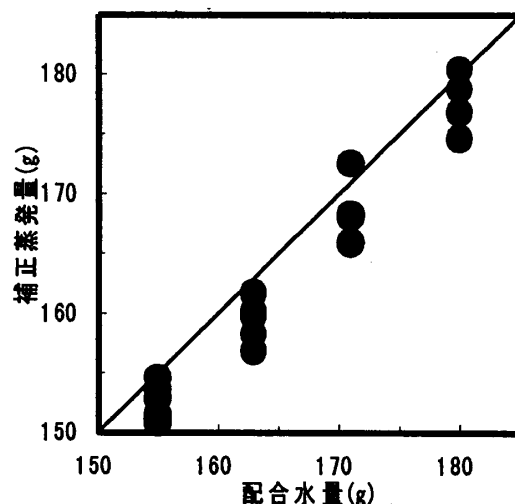
図-7 配合水量と補正蒸発量 (ウェットスクリーンモルタル)
