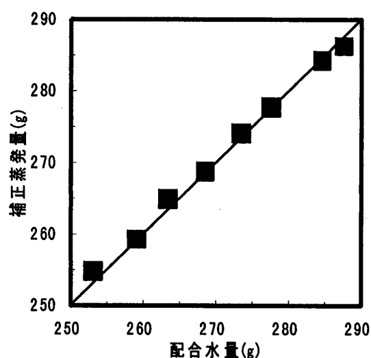
図-3 配合水量と補正蒸発量(モルタル)
