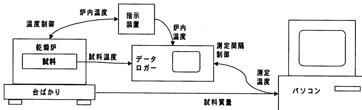
図-1 試験装置
