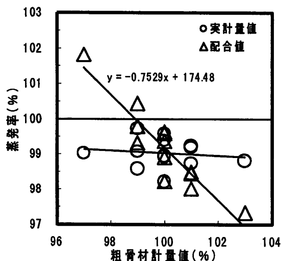
図-8 計量誤差の影響
