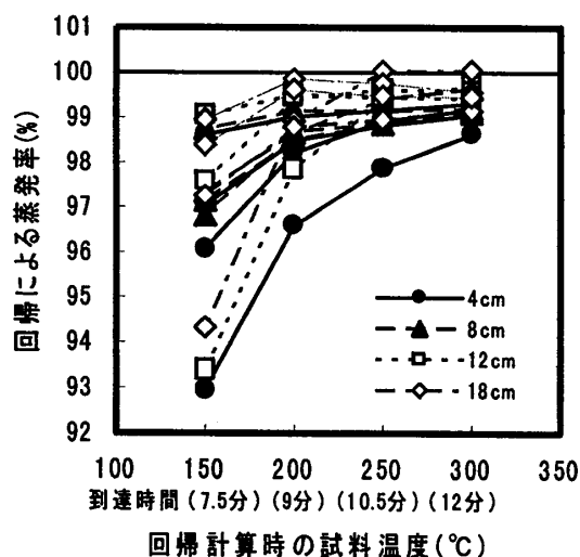
図-14 試料温度と推定蒸発率
