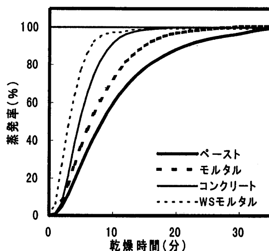
図-10 各試料の乾燥時間と蒸発率の関係
