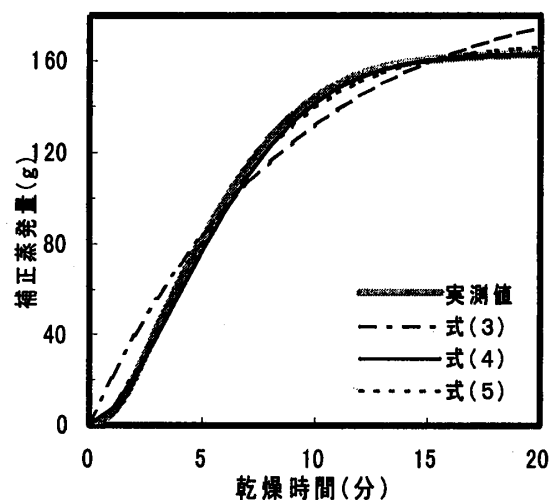
図-12 補正蒸発量と各種回帰曲線
