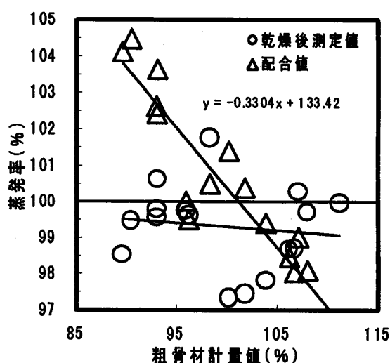
図-9 サンプルング誤差の影響
