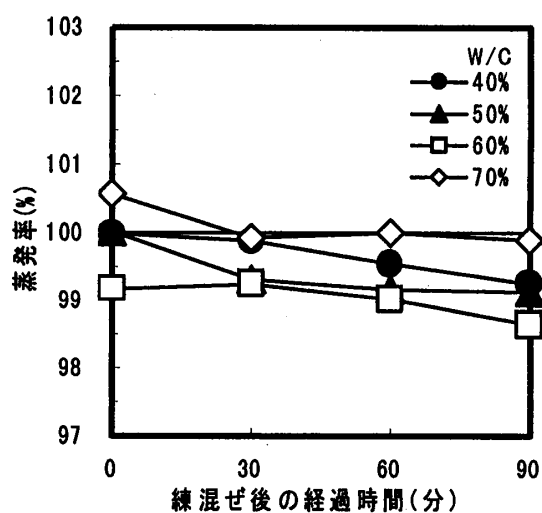
図-5 練混ぜ後の経過時間と 蒸発率(モルタル)
