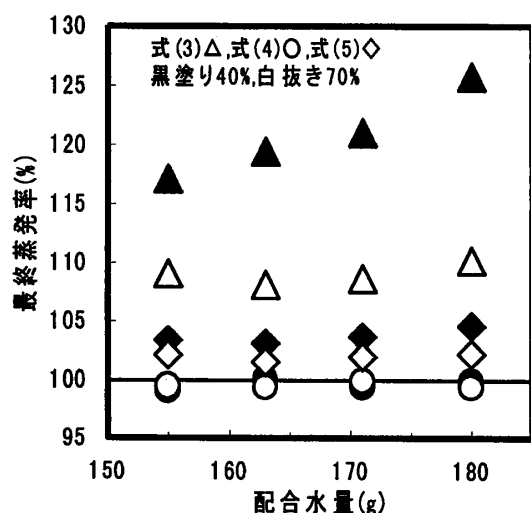
図-13 回帰計算による最終蒸発率
