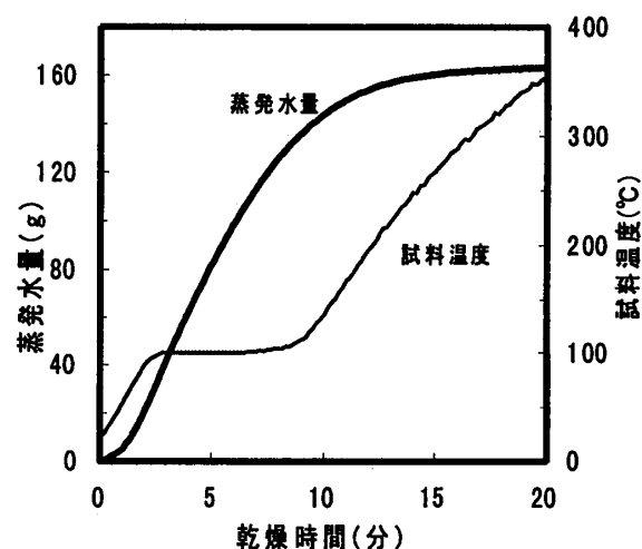
図-11 補正蒸発量と試料温度の関係
