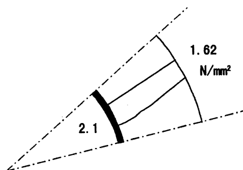
図-6 応力分布図
