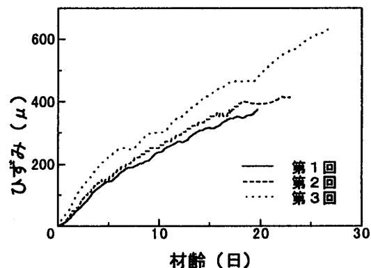
図-8 ひずみの経時変化
