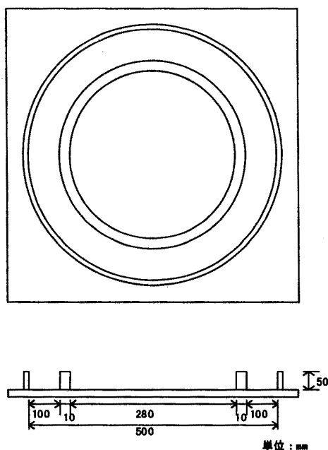
図-5 ドーナツ型拘束枠
