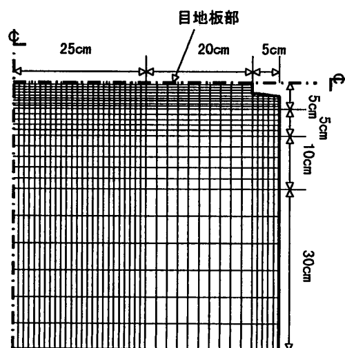
図-3 要素分割図 (Aシリーズ)
