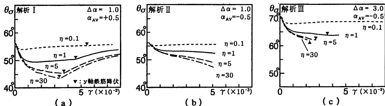
図-4 \theta_\sigma-\gamma 関係
