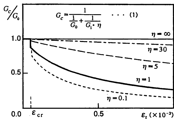
図-2 せん断剛性モデル
