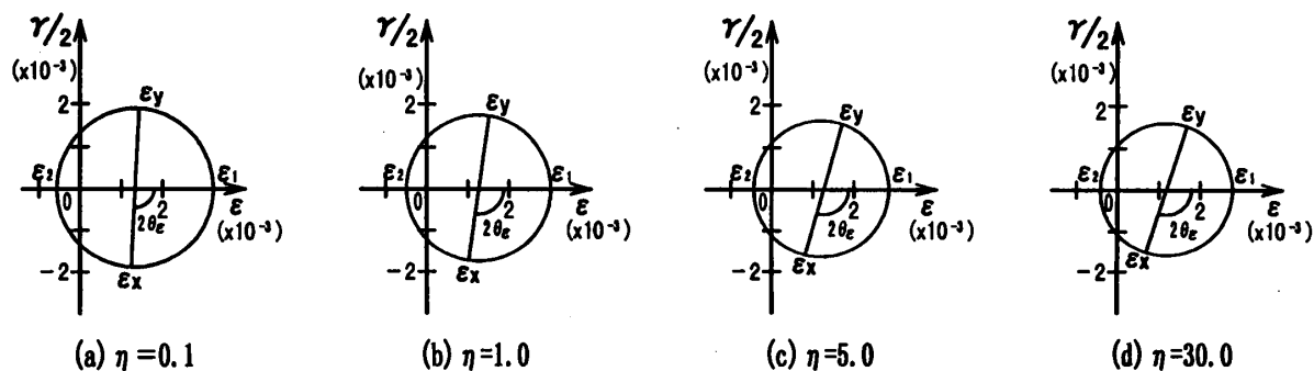
図-6 モールのひずみ円 (解析 I : V=4.0MPa)
