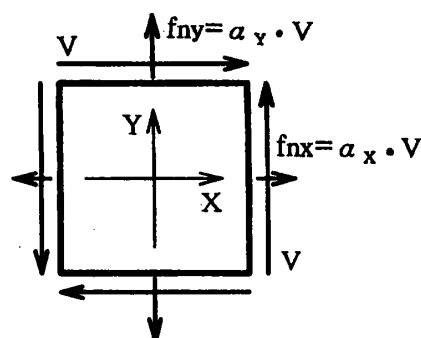
図-1 RC 平板に作用する複合応力
