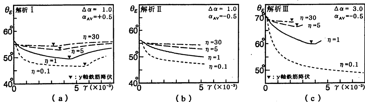
図-5 \theta_\varepsilon-\gamma 関係
