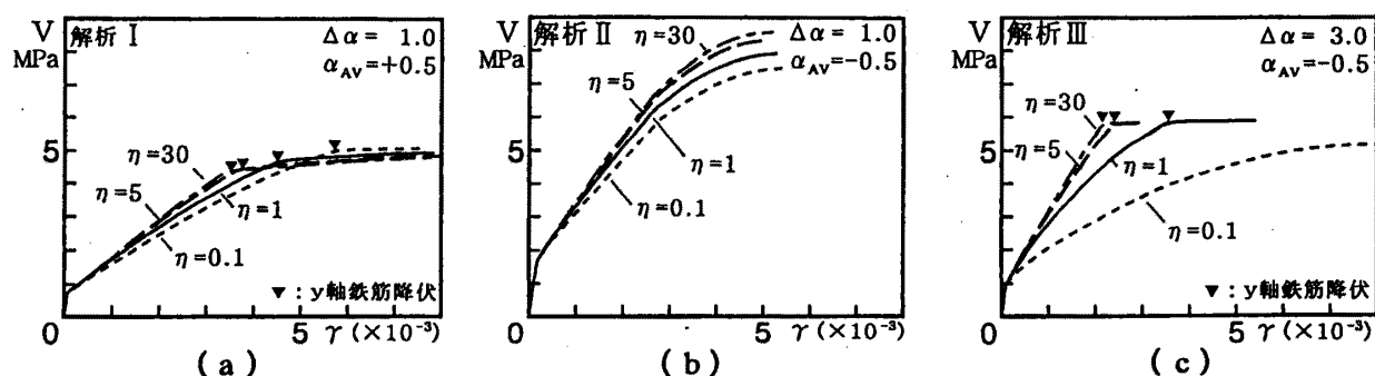
図-3 V-\gamma 関係
