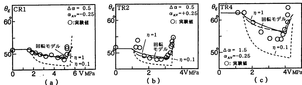
図-9 \theta_\varepsilon-\gamma 関係
