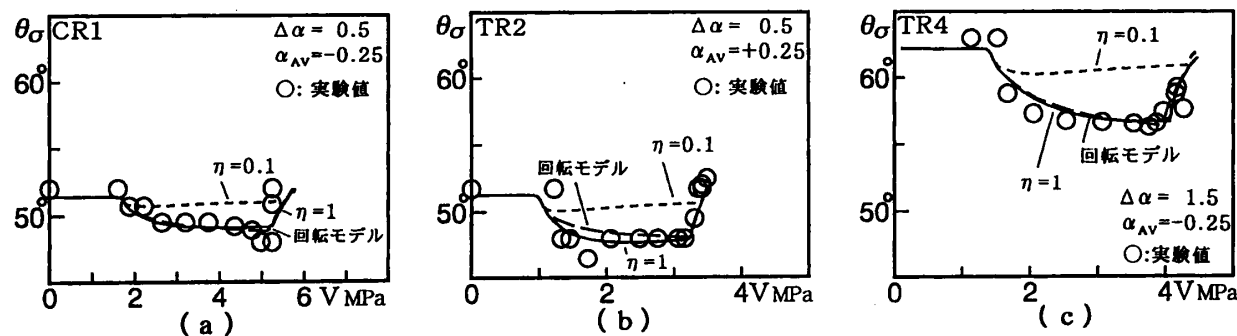
図-8 \theta_\sigma-\gamma 関係
