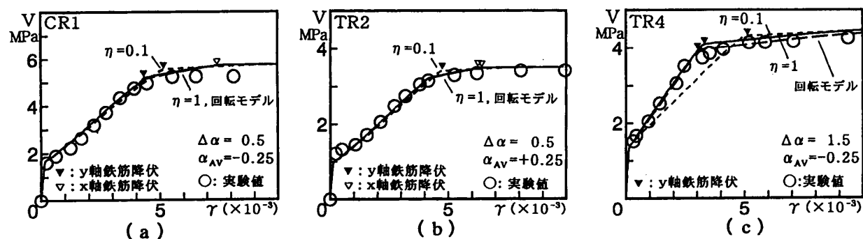
図-7 V-\gamma 関係
