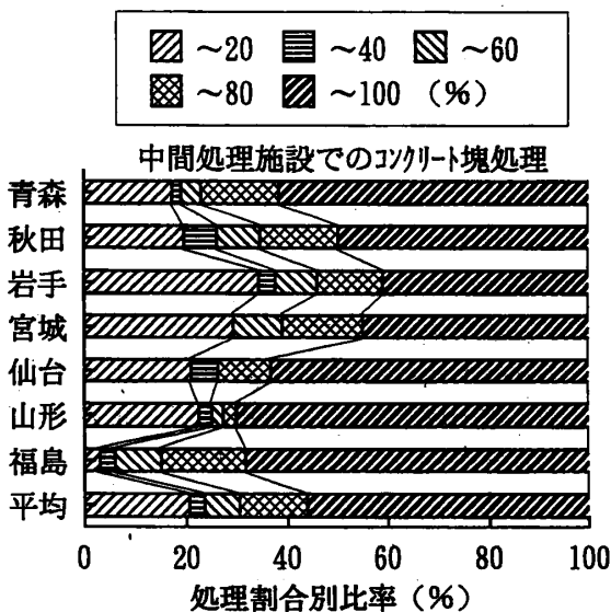
図3 中間処理施設での処理割合
