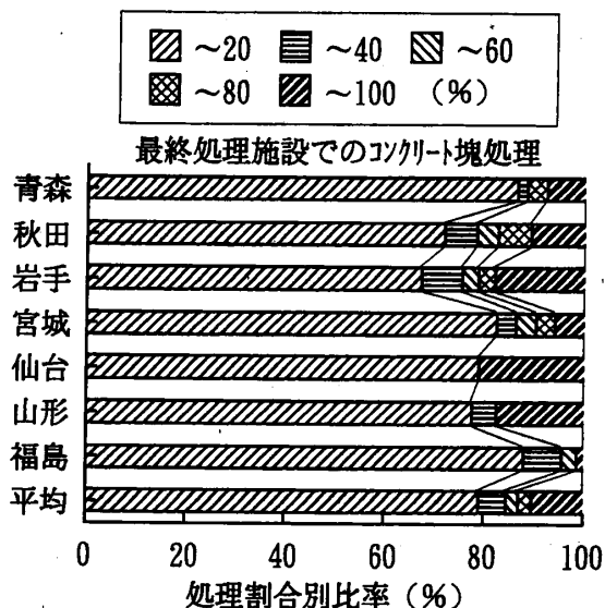
図4 最終処理施設での処理の割合
