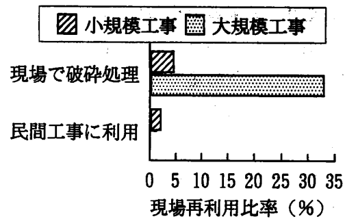
図7 工事規模による現場内再利用
