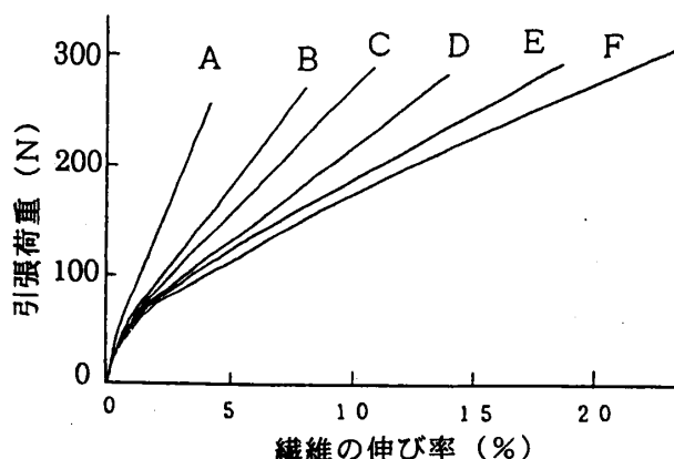
図-1 各種太径ビニロンの物性
