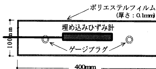
図-1 長さ変化試験用供試体
