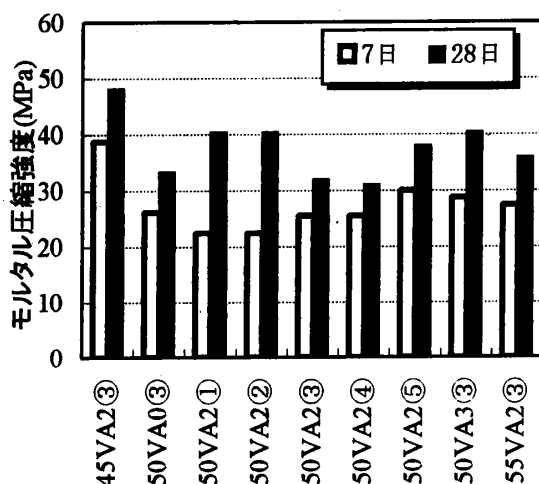
図-2 モルタルの圧縮強度
