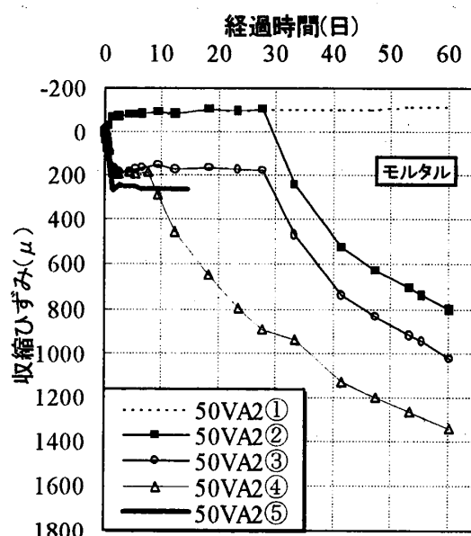
図-5 養生・環境条件が長さ変化に与える影響
