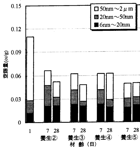
図-8 配合 50VA2 のモルタルの 毛細管空隙分布
