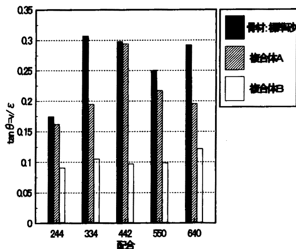
図 - 1 2 配合別体積減少比の比較
