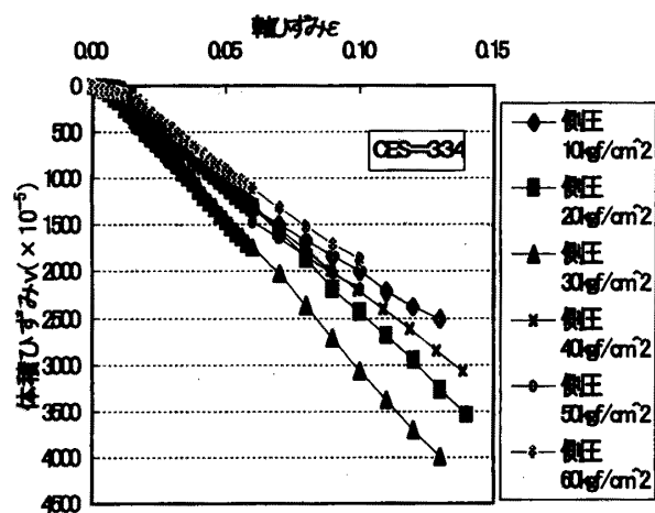
図 - 1 1 軸ひずみ-体積ひずみ曲線
