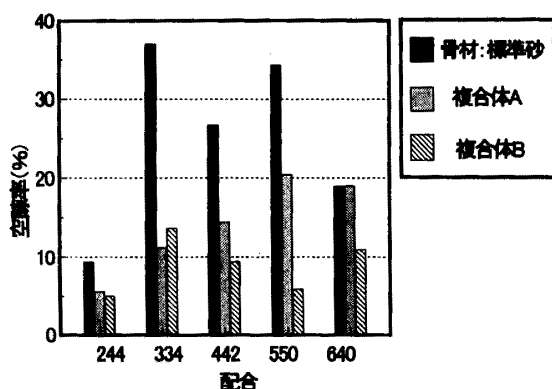
図 - 7 配合別空隙率の比較
