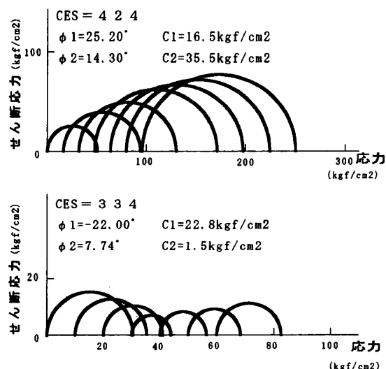
図-1 Mohrの応力円群
