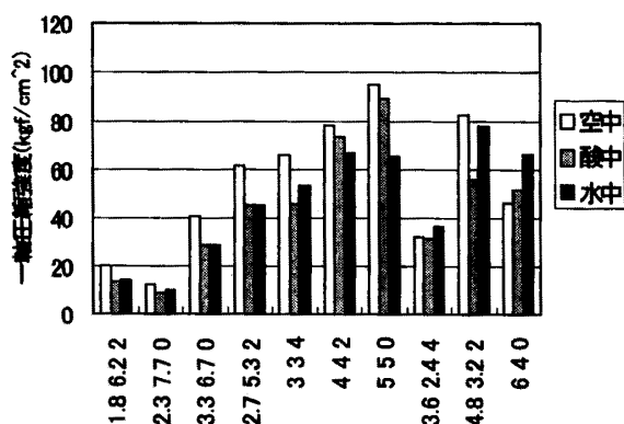
図 - 1 3 配合別一軸圧縮強度の比較
