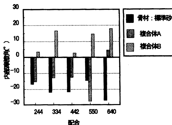
図 - 8 配合別内部摩擦角の比較
