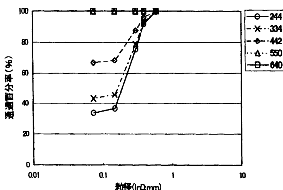
図 - 9 粒度分布 (複合体 A)
