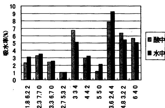
図 - 1 4 配合別吸水率の比較
