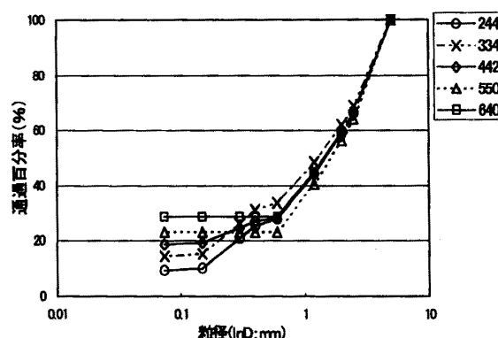
図 - 10 粒度分布 (複合体 B)
