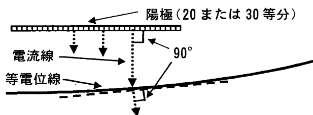
図-4 電流線の作図方法
