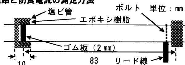
図-2 セル鉄筋
