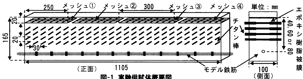
図-1 実験供試体概要図
