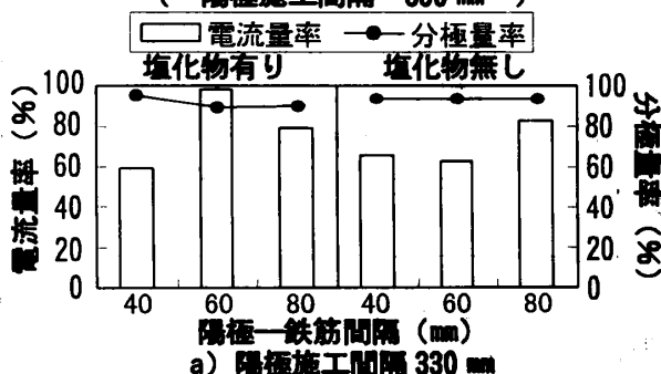
図-12 陽極直下の流入電流量に対する陽極施工範囲外の流入電流量の比率と分極量の比
