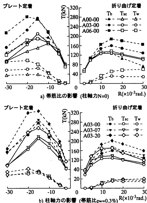
図5 梁主筋引張り力と帯筋・SC部の負担力
