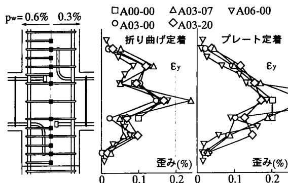
図4 帯筋の歪み分布 ( R=1/67 時)
