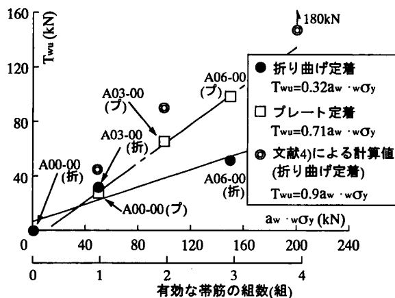
図7 帯筋負担力 T_{wu} - a_w \cdot w\sigma_y 関係
