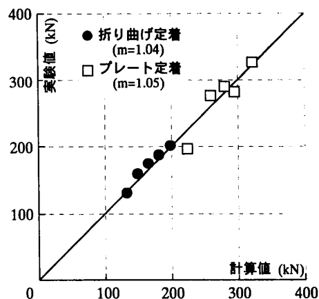
図10 実験値と式(8)(9)による計算値の対応
