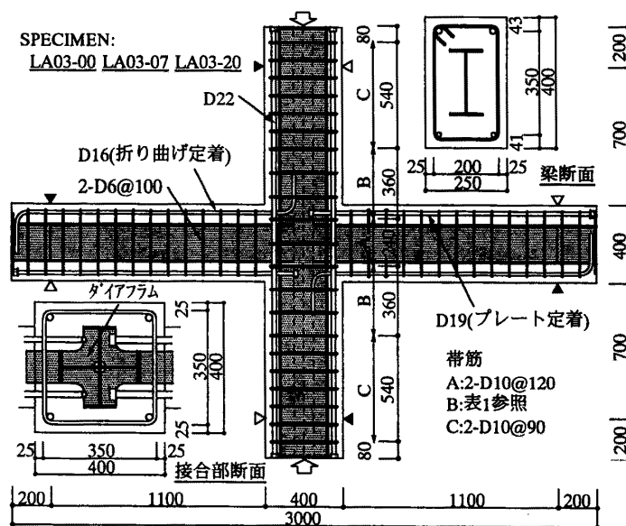
図1 試験体形状および配筋例
