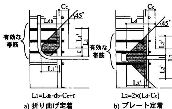
図6 定着に有効な帯筋の仮定
