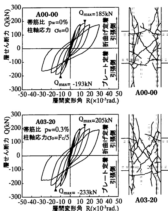
図2 Q-R関係と最終ひび割れ状況
