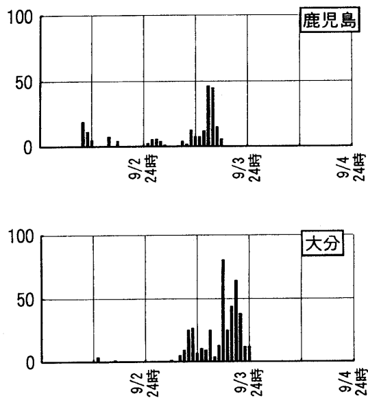
図4 主な地点の時間別降水量 93/09/02 01時～93/09/04 24時
