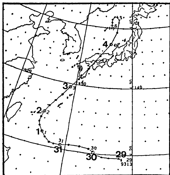
図3 台風9313号の経路 「気象」93年11月号より
